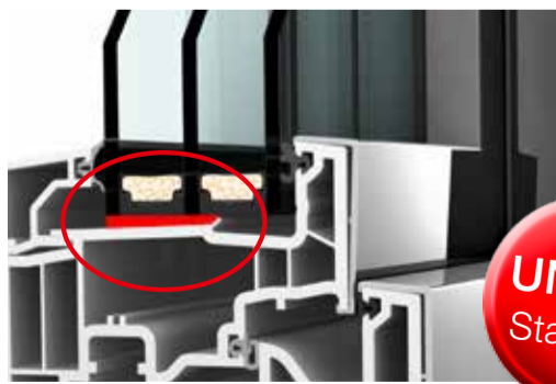
Rundum-Verklebung der Scheibe mit dem Rahmen aushebelsicher und formstabil
