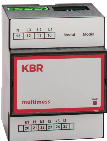
Leistungsmessmodul für die Rückmeldung der aktuellen Leistung von Verbrauchern
