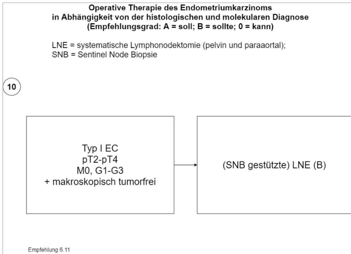
Abbildung 11: Handlungsleitenden Algorithmen 1-10
