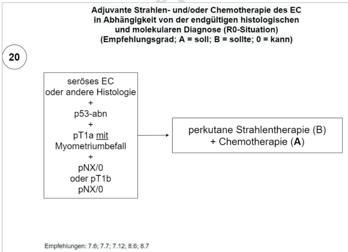
Abbildung 12: Handlungsleitende Algorithmen 11-20
