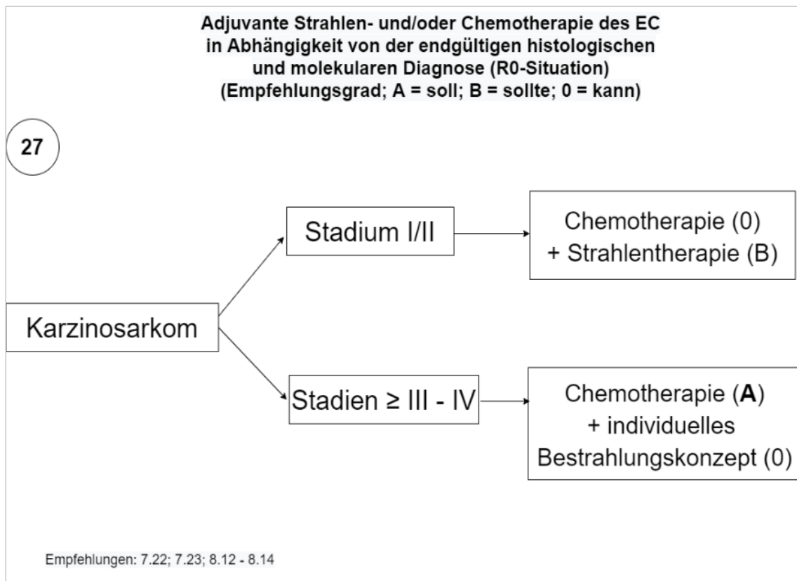
Abbildung 13: Handlungsleitende Algorithmen 20-27
