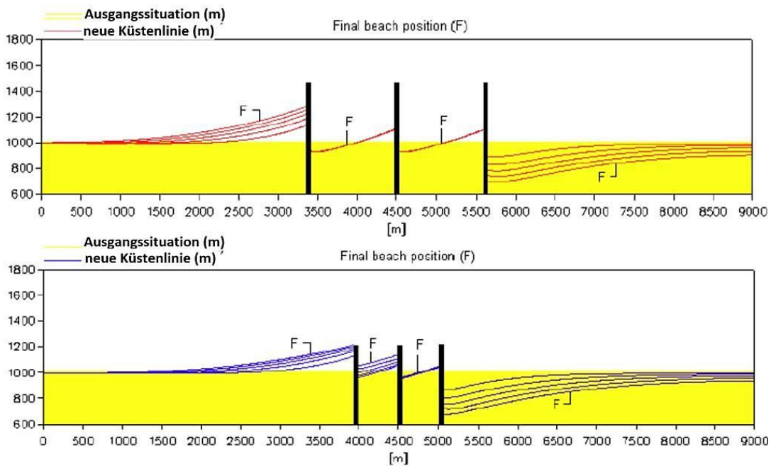
Abb. 8: Bühnenfeld (verändert nach MANGOR et. al 2017)
