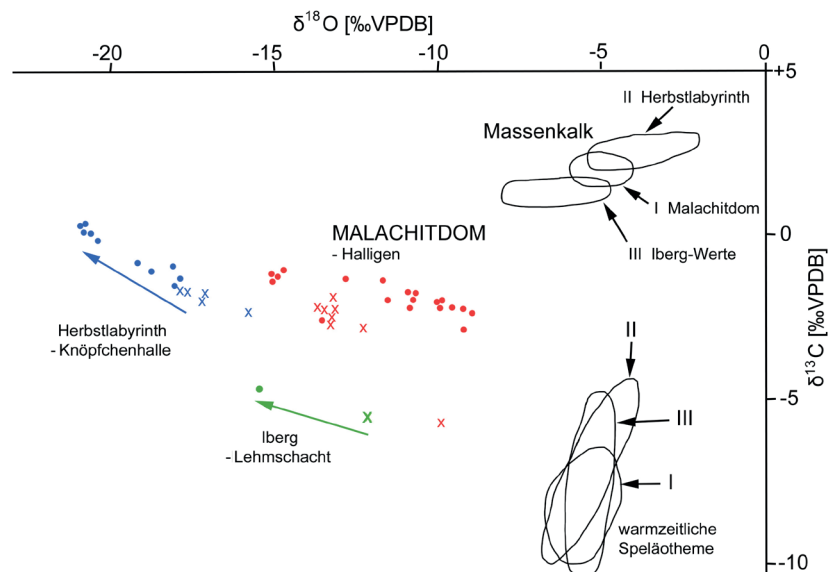
Abb. 7: C/O-Isotopenzusammensetzung der Umbrellacalcite (x - Stiele, ● - Schirme) des Malachitdomvorkommens im Vergleich zu Äquivalenten des Herbstlabyrinths (Knöpfchenhalle - neue Daten) und dem Lehmschacht (Iberg/Harz). Die Felder für die mittel/oberdevonischen Massenkalke (Wirtsgesteine) und die warmzeitlichen Speläotheme der Höhlen sind der Literatur entnommen (I - Malachitdom nach Richter & Riechelmann (2008); II - Herbstlabyrinth/Breitscheid nach Richter et al. 2010,2011; III - Lehmschachthöhle Iberg/Harz nach Richter et al. 2017a)
