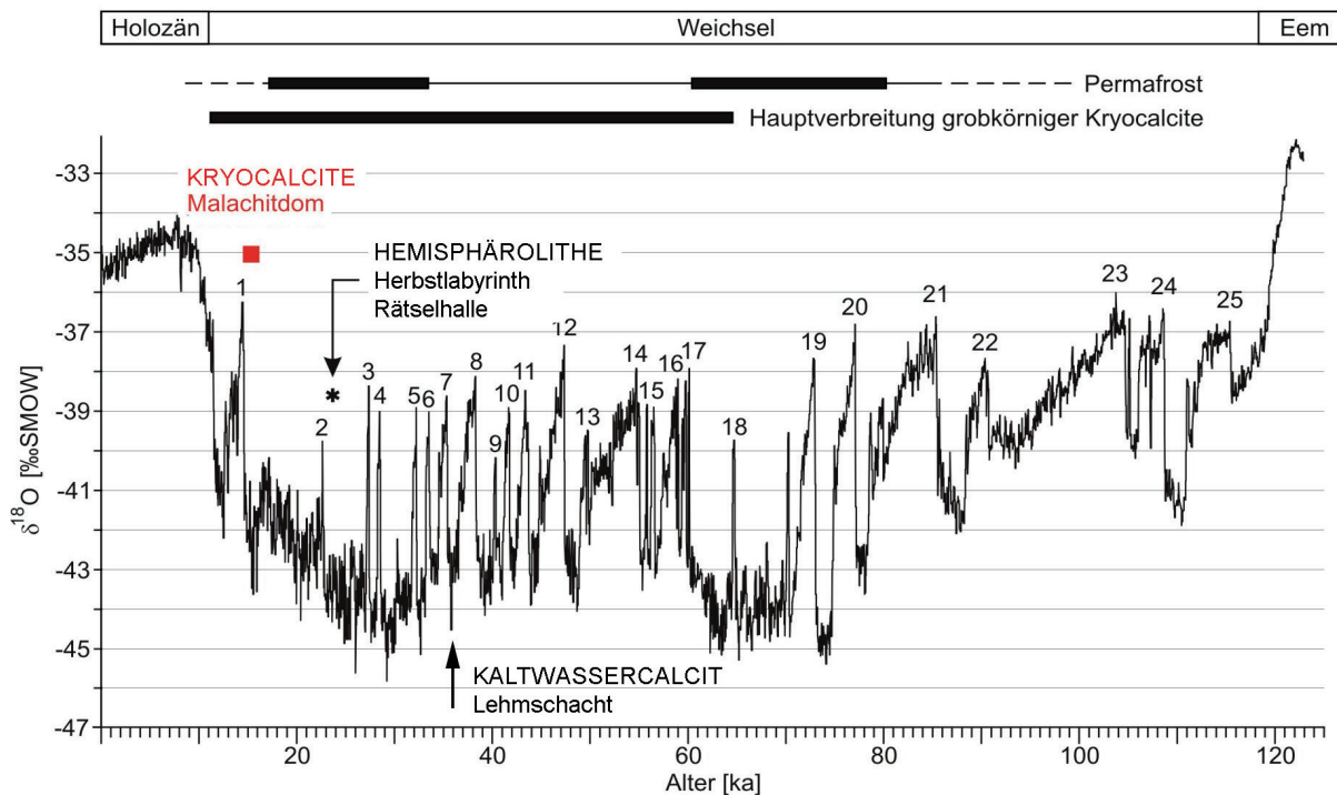
Abb. 9: Korrelation der ^{230}\text{Th}/\text{U} -Datierungen der Umbrellacalcite (neue Daten) sowie von Cupulasphärolithen (Richter & Riechelmann 2008) des Malachitdoms, von Kaltwassercalciten des Lehm-schachts (Iberg/Harz nach Richter et al. 2017a) sowie Hemisphärolithen der Rätselhalle (Herbstlabyrinth/Breitscheid - neue Daten) im Vergleich zur \delta^{18}\text{O} -Kurve des NGRIP-Eisbohrkerns (North Greenland Ice Core Project Members 2004). Gleich bezifferte Stadiale folgen immer jeweils den Interstadialen. Zeitspannen kontinuierlichen (dicke Linien) und diskontinuierlichen (dünne Linien) Permafrosts nach Liedtke (1993) und Vandenberghe & Pissart (1993).
