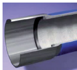
Einsteckschweißmuffe mit Anschlagring im Muffengrund
