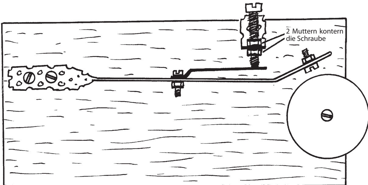
fertiger Unterbrecher-Kontakt
