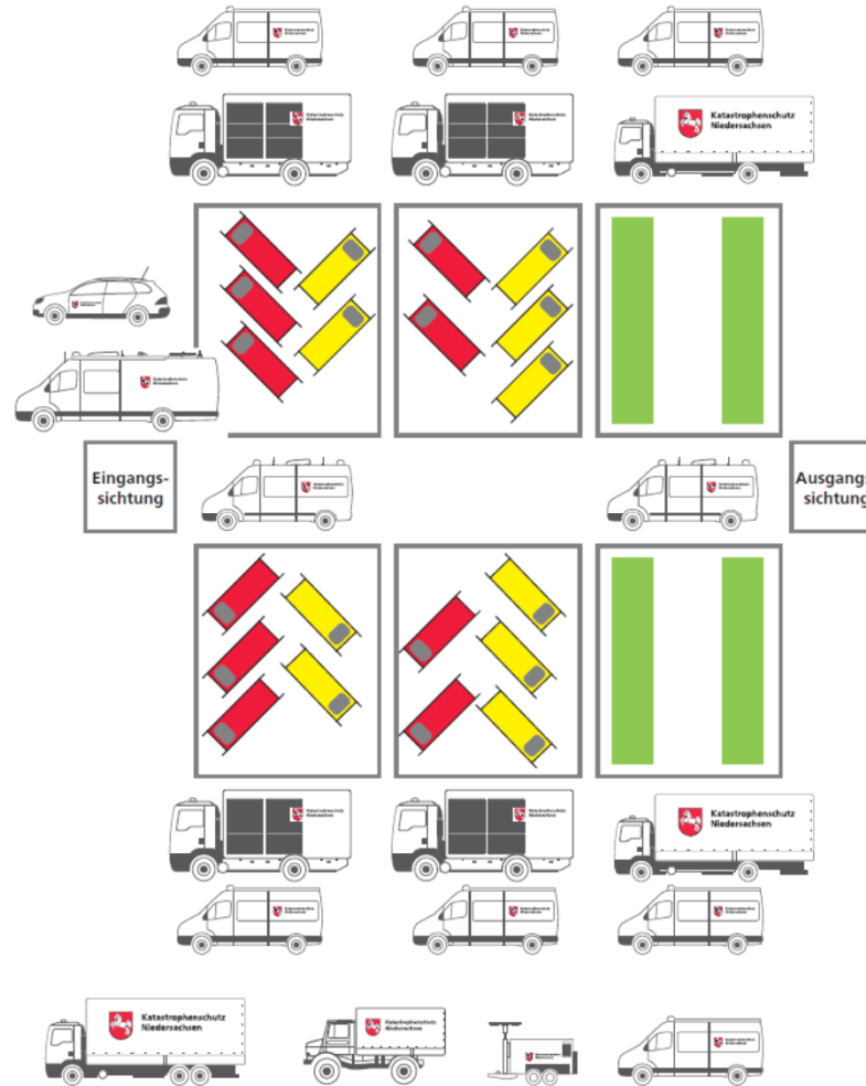
Übersicht BHP 50 mit Fahrzeugen
