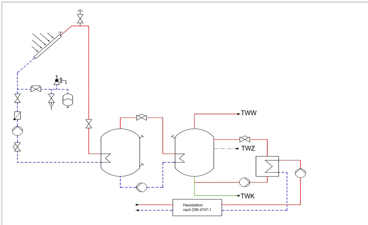
Abbildung 20: Solaranlage mit Pufferspeicher und Trinkwassererwärmer mit außen liegenden Wärmeübertrager für die Nachheizung mit Fernwärme
