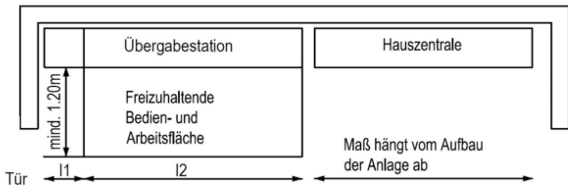
Abbildung 6: Bsp. Hausanschlusswand
