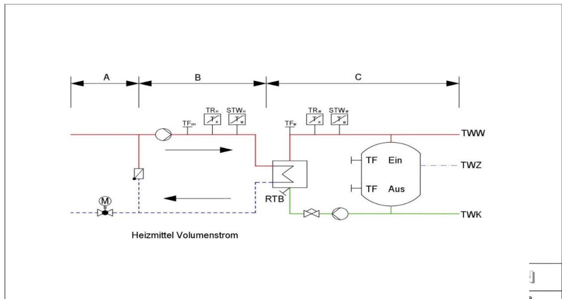
Abbildung 17: Direkteingebundenes Speicherladesystem vorgeschaltet wird eine UEST gemäß Schema in Kapitel 5.1
