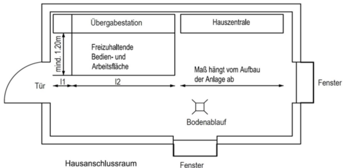
Abbildung 5: Bsp. Hausanschlussraum
