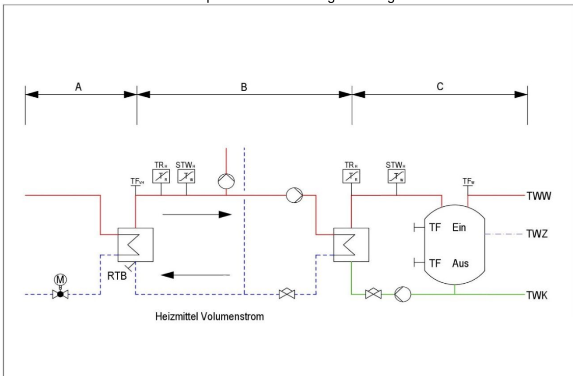
Abbildung 13: Hauszentrale Trinkwassererwärmung Prinzipschemas für die Hauszentrale, diese erhebt keinen Anspruch auf Abdeckung aller möglichen Varianten.
