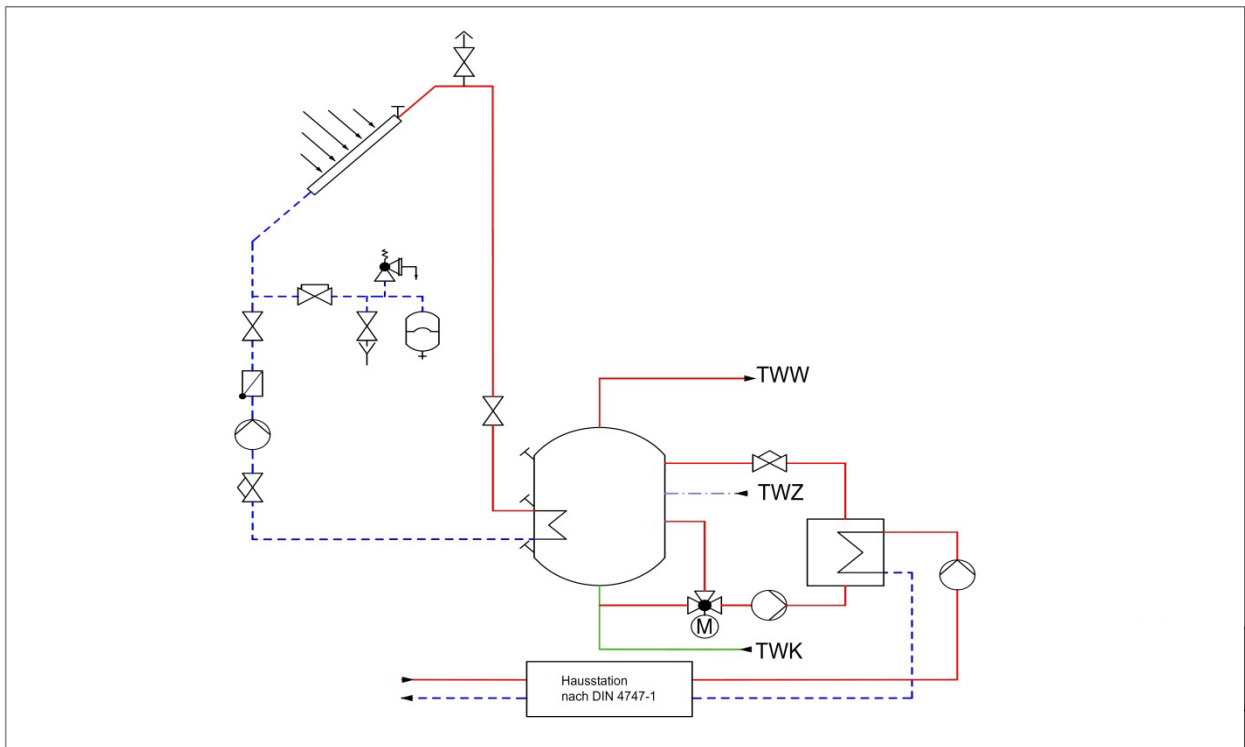
Abbildung 19: Trinkwassererwärmer mit außen liegendem Wärmetauscher für die Nachheizung
