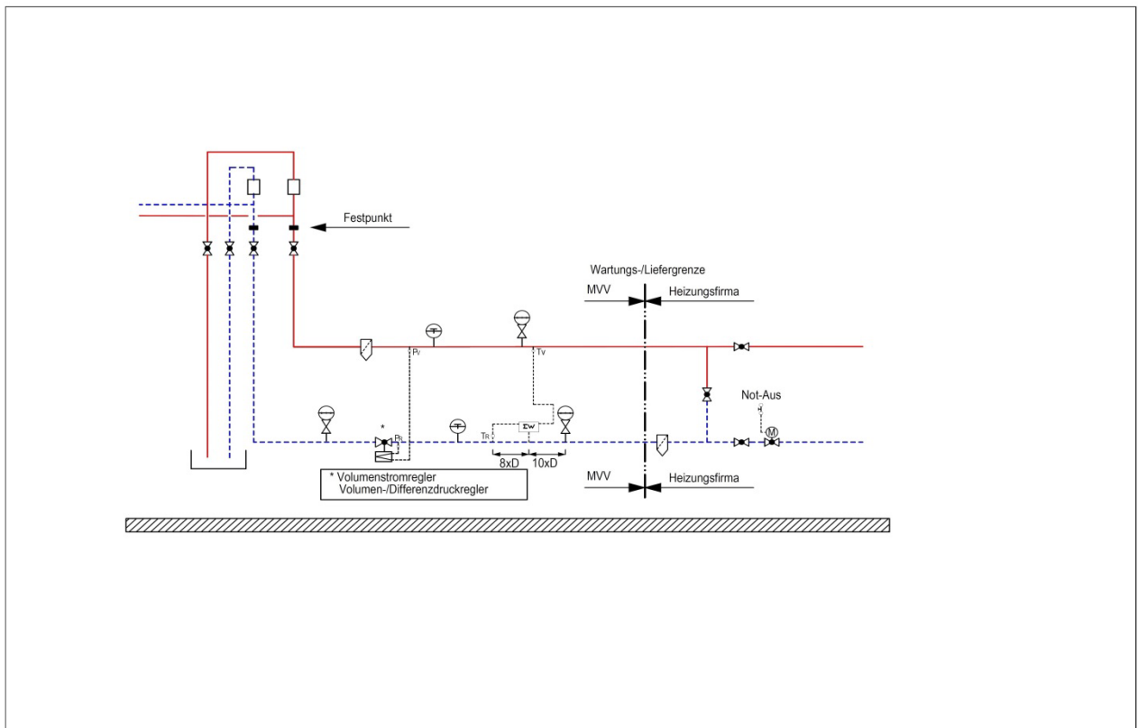
Abbildung 7: Schema Übergabestation (UEST)
