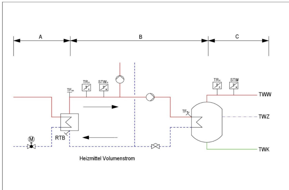
Abbildung 11: Hauszentrale Trinkwassererwärmung Prinzipischemas für die Hauszentrale, diese erhebt keinen Anspruch auf Abdeckung aller möglichen Varianten.
