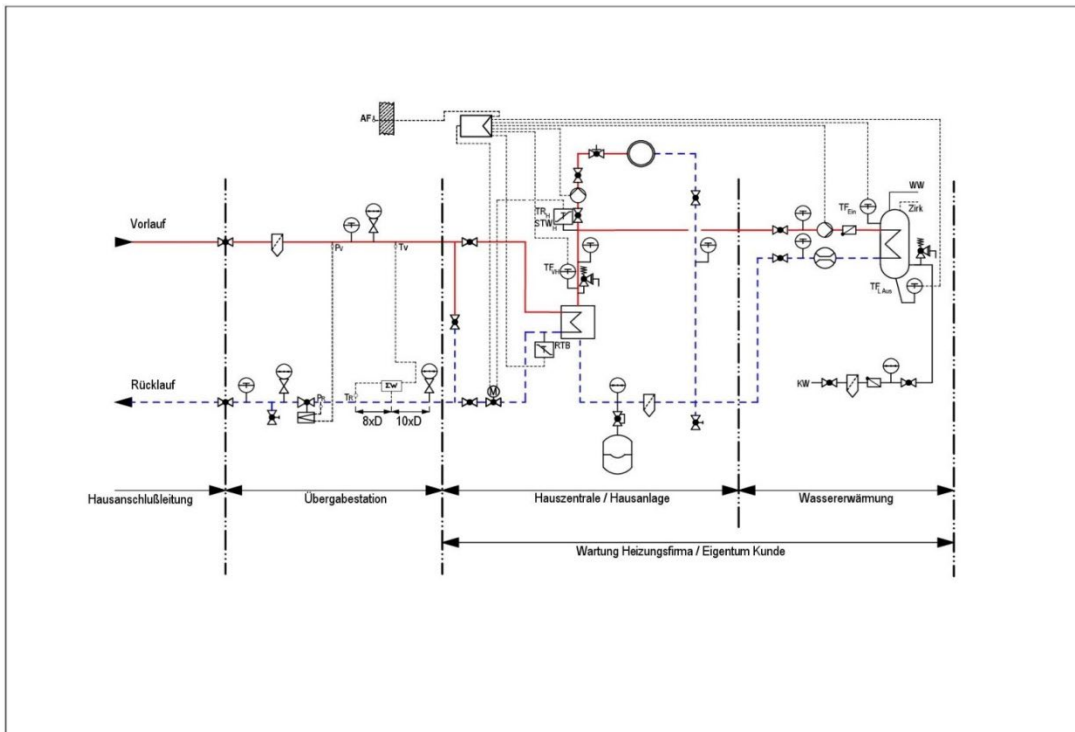
Abbildung 9: Schema Übergabestation (UEST) und Hauszentrale mit Trinkwassererwärmung
