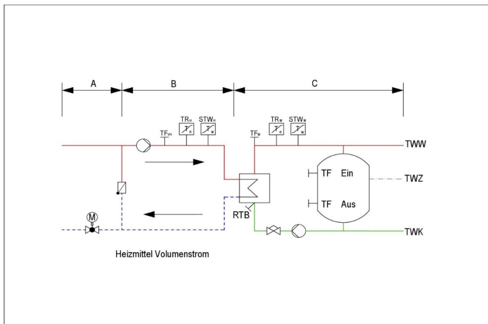
Abbildung 12: Hauszentrale Trinkwassererwärmung Prinzipischemas für die Hauszentrale, diese erhebt keinen Anspruch auf Abdeckung aller möglichen Varianten.
