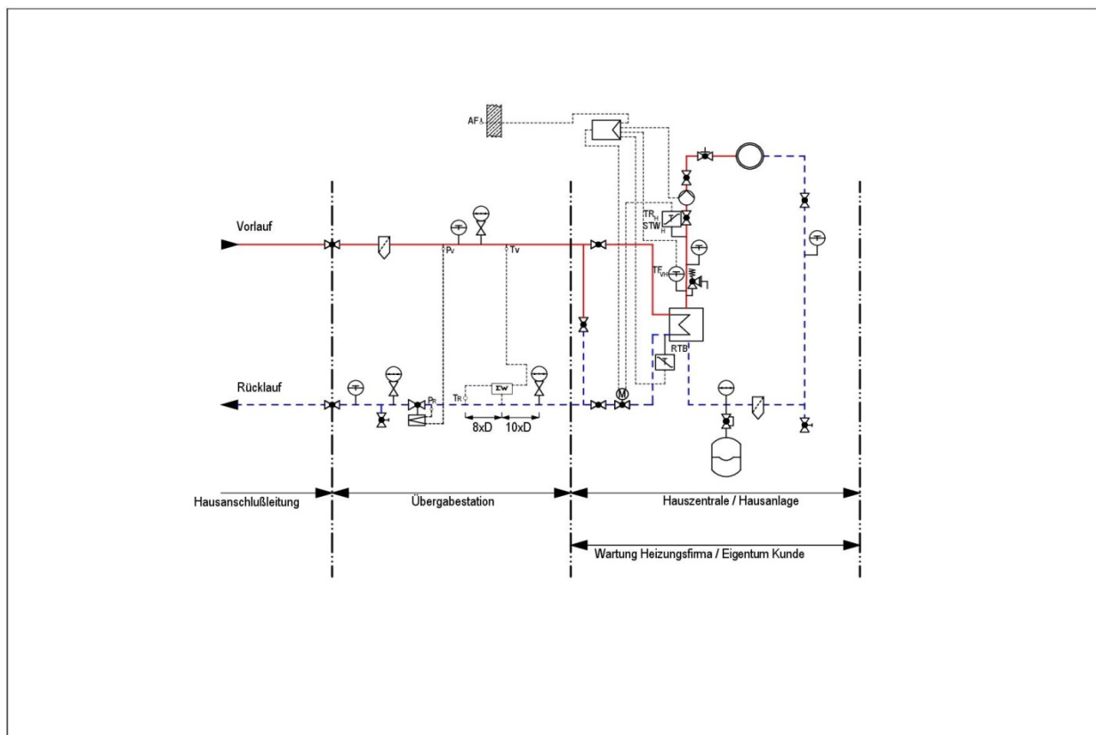
Abbildung 10: Übergabestation und Hauszentrale-Raumheizung für den indirekten Anschluss
