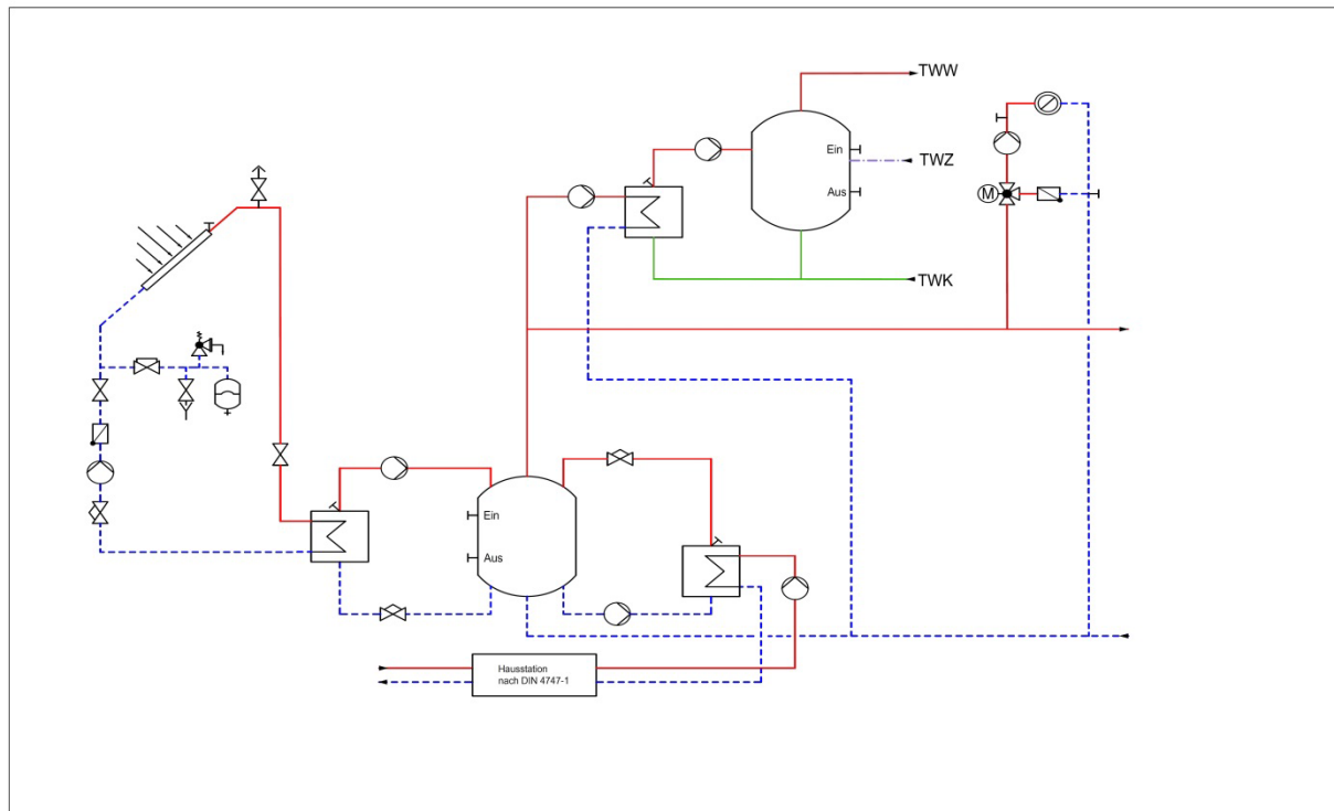
Abbildung 21: Solar unterstützten Heizsystems, Pufferspeicher mit außen liegenden Wärmeübertragern für die Solaranlage und die Nachheizung mit Fernwärme
