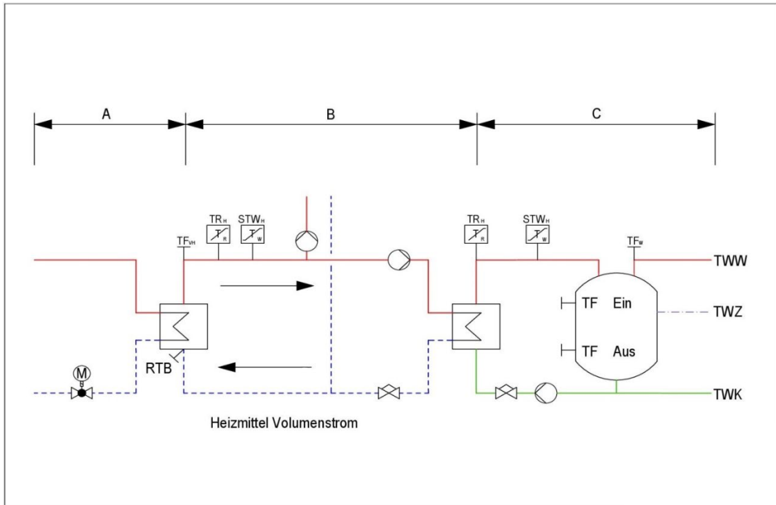
Abbildung 13: Hauszentrale Trinkwassererwärmung Prinzipschemas für die Hauszentrale, diese erhebt keinen Anspruch auf Abdeckung aller möglichen Varianten.
