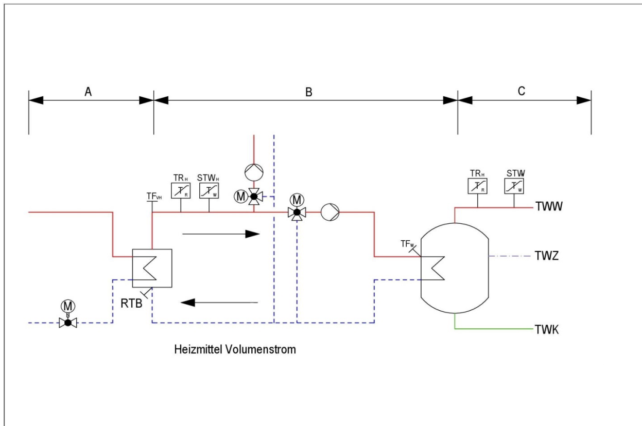
Abbildung 15: Hauszentrale Trinkwassererwärmung Prinzipschemas für die Hauszentrale, diese erhebt keinen Anspruch auf Abdeckung aller möglichen Varianten.
