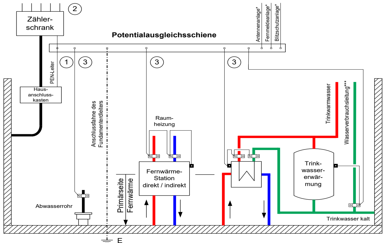
Abbildung 3: Beispiel eines Potenzialausgleichs
