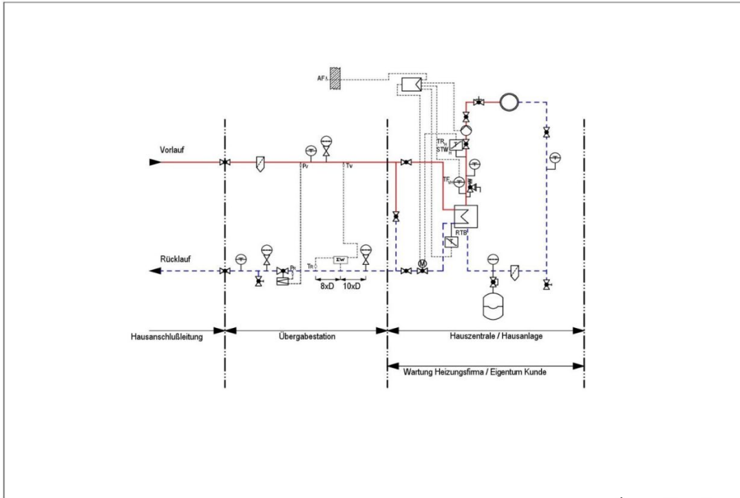
Abbildung 8: Schema Übergabestation (UEST) und Hauszentrale
