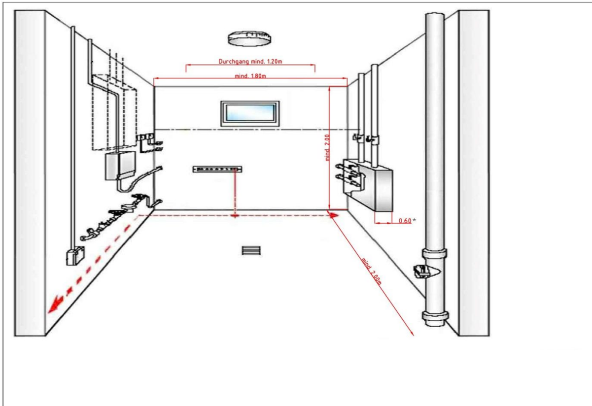
Abbildung 4: Schematische Darstellung eines Hausanschlussraums für eine UEST / KHST. Die angegebenen Maße -sind die Mindestmaße- die einzuhalten sind. Maß kann je nach Stationstyp in der Tiefe variieren
