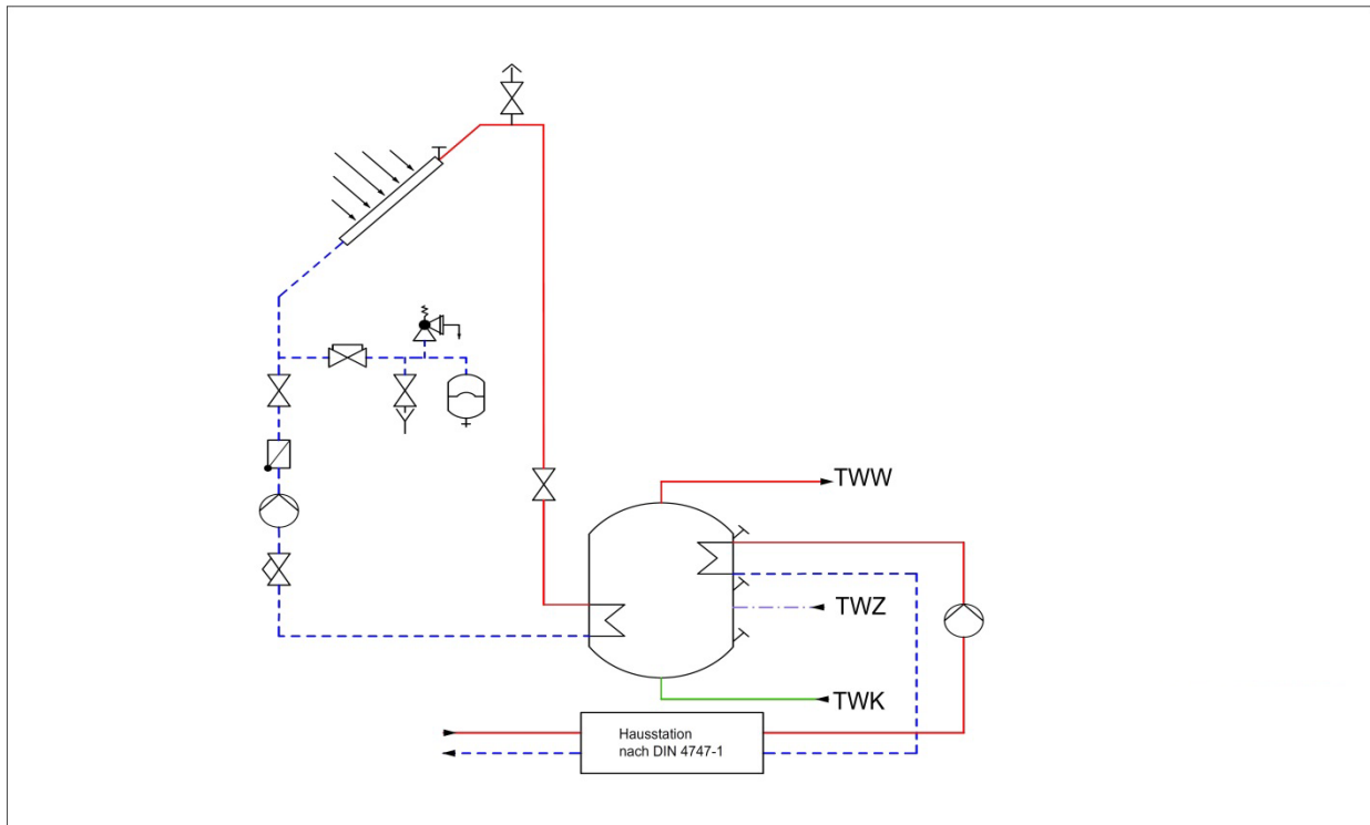
Abbildung 18: Speicher mit innenliegender Heizfläche für Solar und Fernwärme
