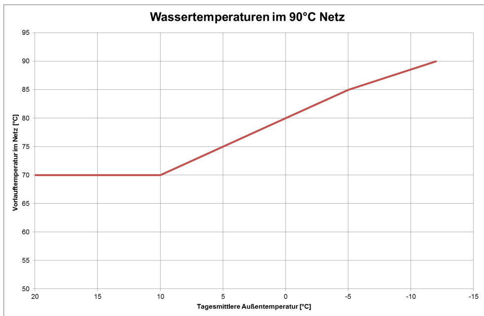
Abbildung 1: Netzvorlauftemperatur T_v in Abhängigkeit von der Außentemperatur T_a ; bei einer gleitend-konstanten Fahrweise
