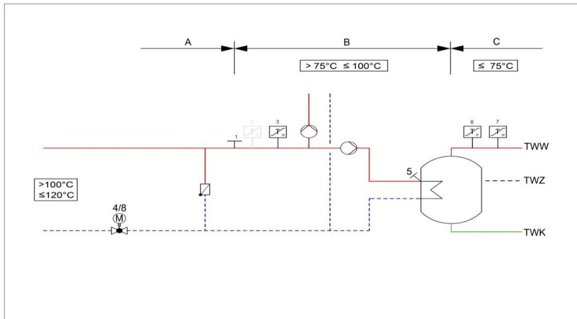
Abbildung 16: Erforderliche sicherheitstechnische Ausrüstung nach Zeile 2 grau dargestellte Komponenten nicht erforderlich
