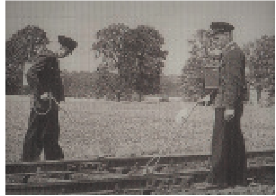
Bild 28: Laschenkammerprüfung mit „MATISA-Sonirail“
