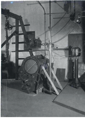
Bild 13: Durchstrahlung eines reparaturgeschweißten Grauguss-Lokzylinders
