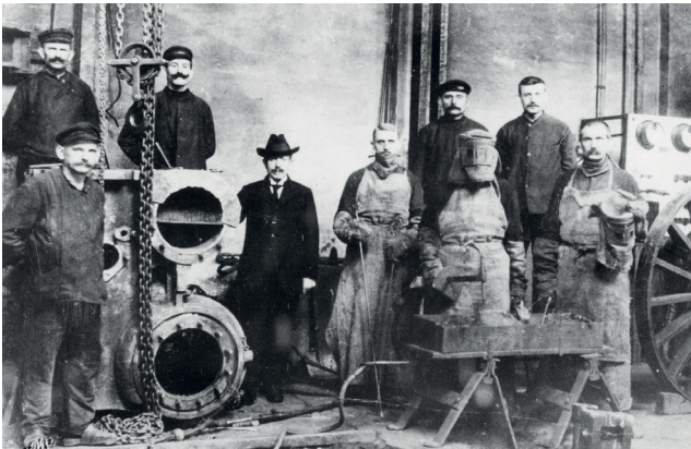
Bild 2: Lichtbogen-Grauguss-Warmschweißerei des Ausbesserungswerkes Wittenberge um 1916
