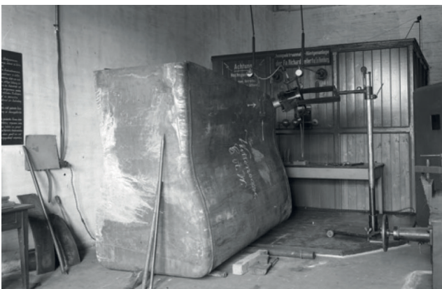
Bild 16: Durchstrahlung einer geschweißten kupfernen Lok-Feuerbüchse im Röntgenlabor
