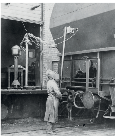
Bild 10: Untersuchung der Schweißnähte an einem Schüttgutwagen
