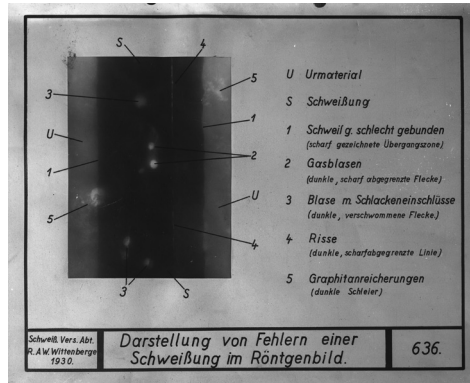
Bild 14: Darstellung von typischen Schweißnahtfehlern auf einem Röntgenfilm
