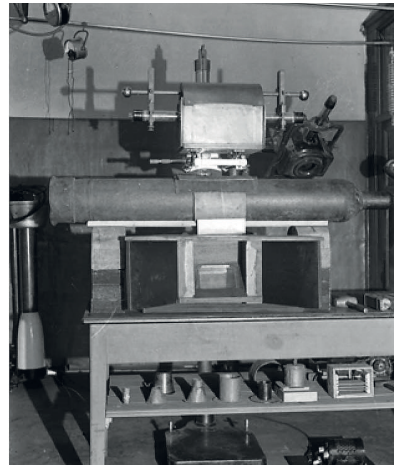
Bild 9: Druckgasflaschen-Prüfstand mit Leuchtschirm
