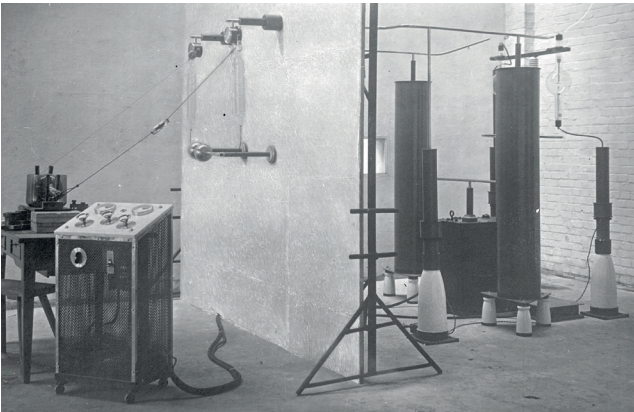
Bild 8: Stationäre Hochleistungs-Röntgenanlage der Firma R. Seifert & Co. Hamburg
