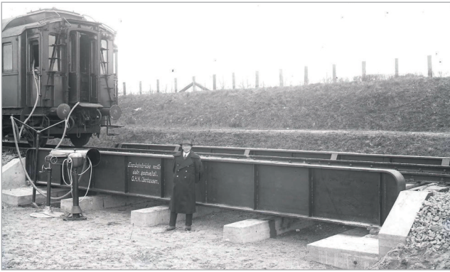
Bild 18: Carl Kantner und der fahrbare Röntgenprüfwagen beim Prüfen der ersten voll geschweißten Eisenbahnbrücke in Oberhausen um 1930
