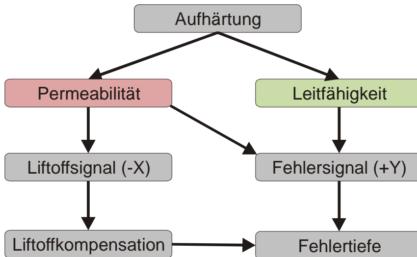
Abbildung 3: Einfluss der Aufhärtung auf die Fehlertiefenbestimmung
