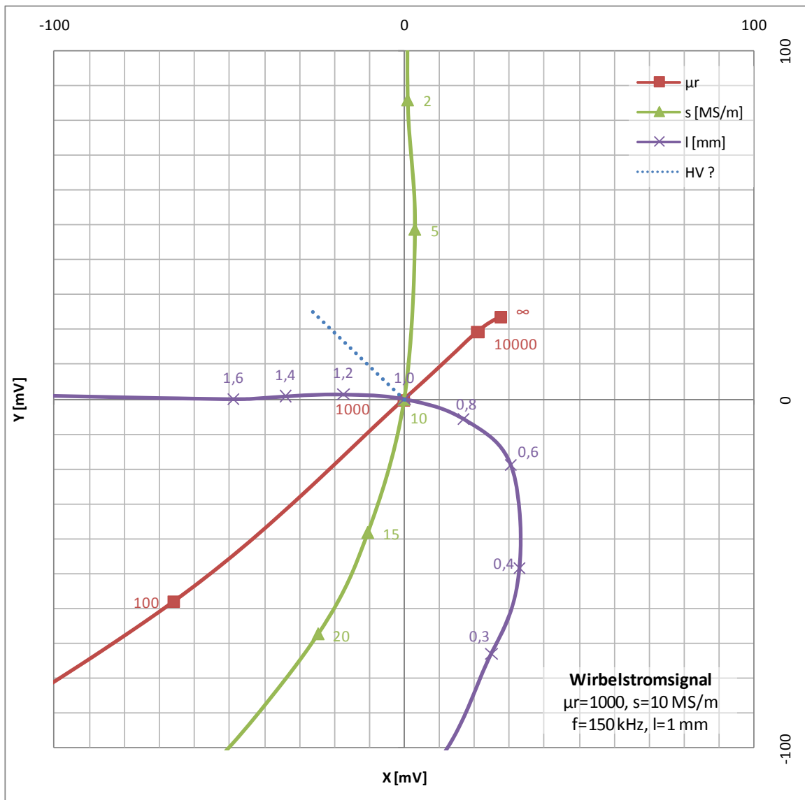
Abbildung 2: Wirbelstromsignal in der komplexen Ebene (XY-Anzeige)
