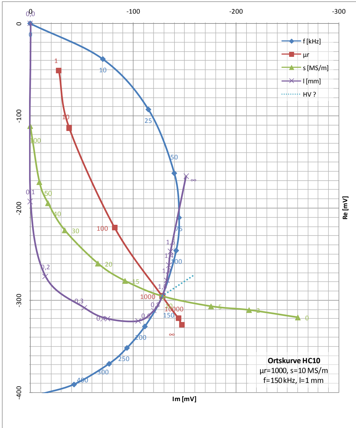
Abbildung 1: Berechnete Ortskurven der Wirbelstromsonde HC10
