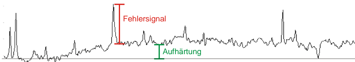
Abbildung 4: Reale Messdaten in YT-Darstellung
