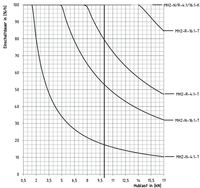
Einschaltdauerdiagramm MH2
