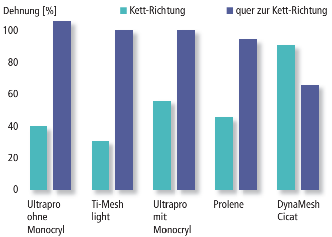
Abbildung 2 Uni-axiale Prüfung der Netze auf Stabilität und Dehnbarkeit in Relation zum Verlauf der Kettfäden. 4 x 8 cm Streifen (bis zur Ruptur in % von der Ausgangslänge), einmal nach Zuschnitt der Streifen in Kettrichtung, und einmal nach Zuschnitt der Streifen quer zur Kettrichtung. a _Maximale Reißkraft bis zur Ruptur, b _Maximale Dehnbarkeit.
