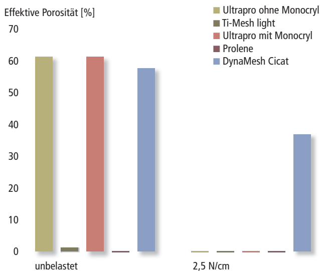
Abbildung 5 Bestimmung der effektiven Porosität nach Mühl [2] in Ruhe und unter Belastung in Richtung der Hauptdehnbarkeit.
