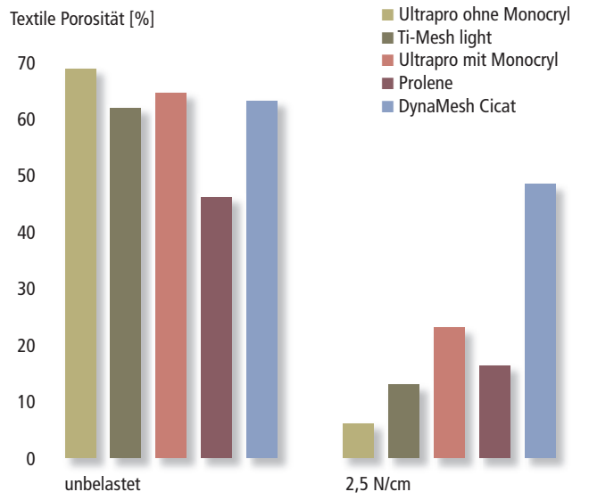
Abbildung 3 Bestimmung der textilen Porosität als Fläche aller Poren, sowohl in Ruhe als auch unter Zugbelastung in Richtung der Hauptdehnbarkeit.
