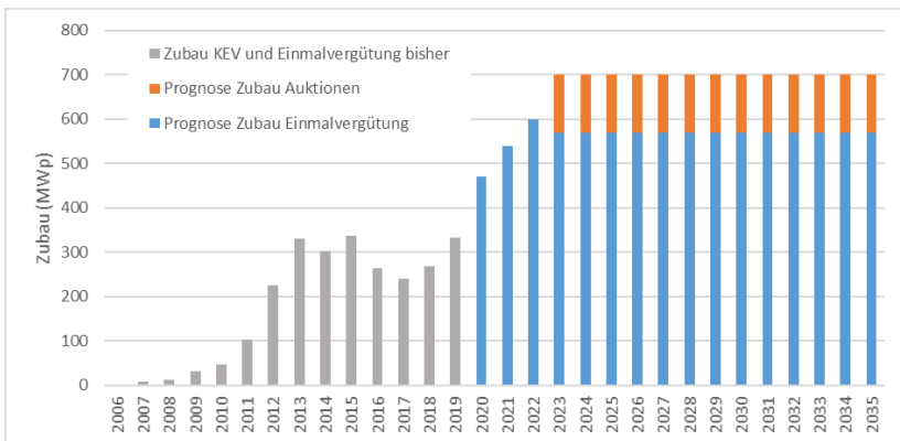
Abbildung 3: Bisheriger und prognostizierter Zubau der Photovoltaik in der Schweiz
