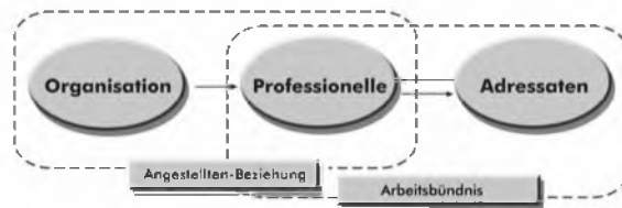
Abbildung 1: Doppeltes-Prinzipal-Agent-Modell
