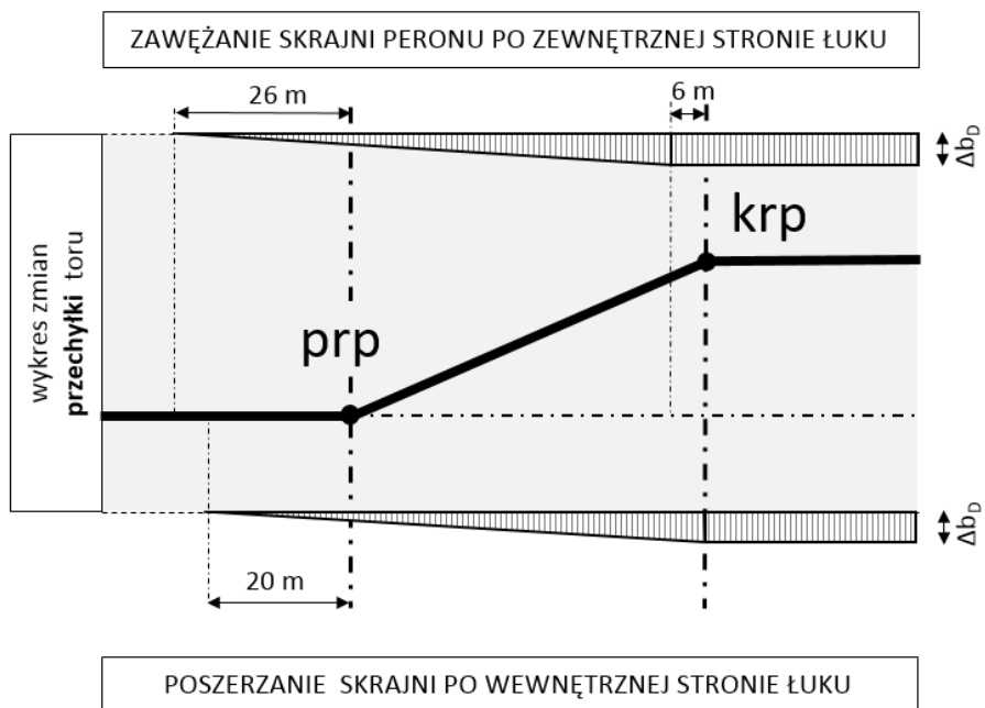
Rysunek nr 5 Zasady zmian poszerzeń i zwężeń skrajni Granicznej Skrajni Zabudowy z uwagi na zmiany przechyłki toru
