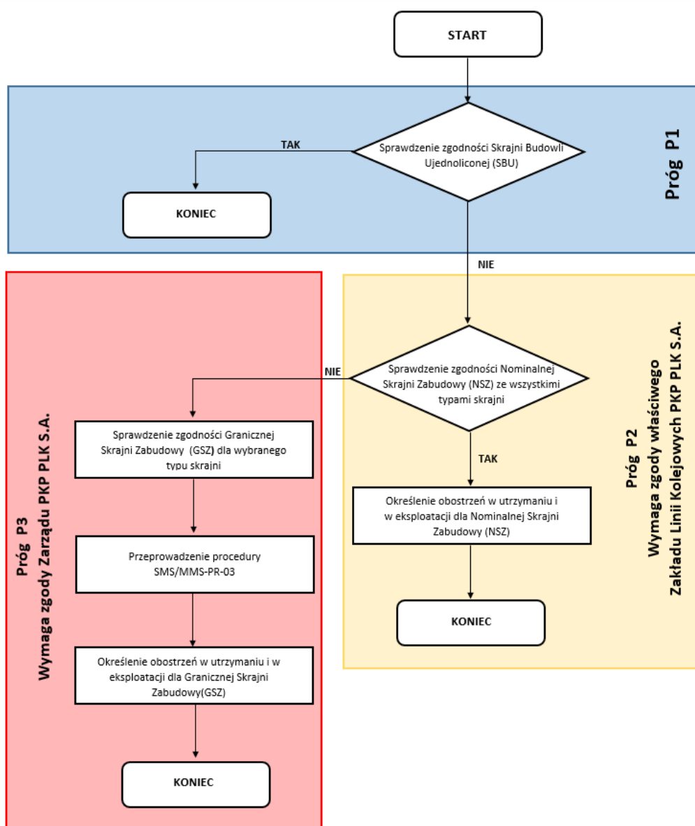
Rysunek nr 1 Schemat postępowania w przypadku niezachowania Skrajni Budowli Ujednoliconej (SBU)
