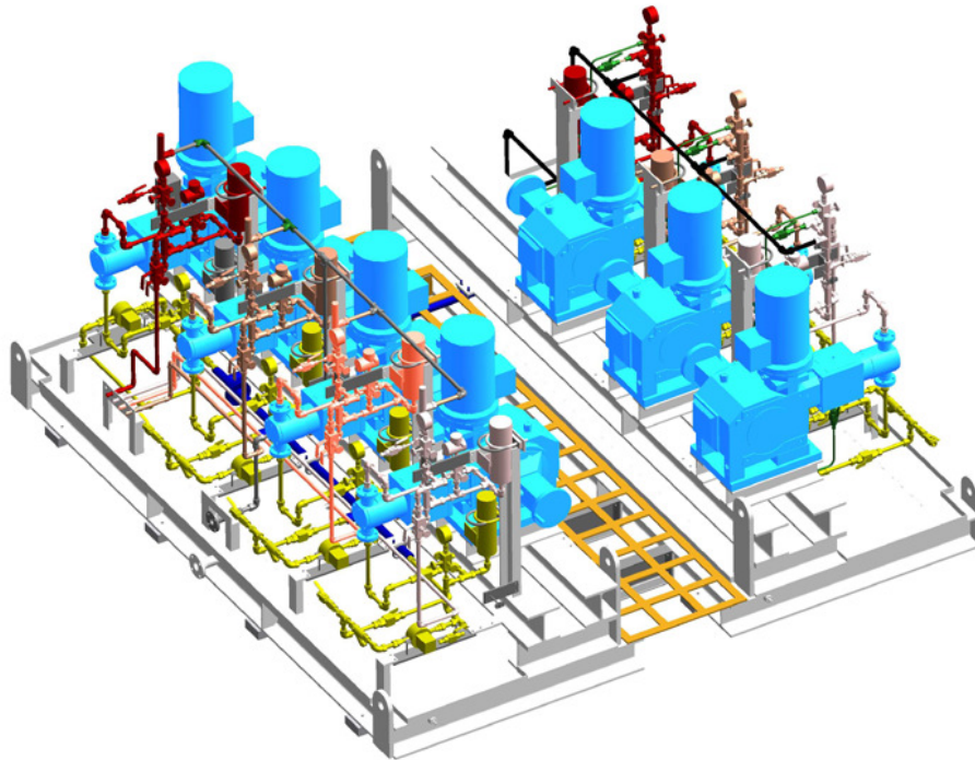
Das Bild zeigt: Dosieranlage zur Methanol-Injektion für die Öl- und Gasindustrie
