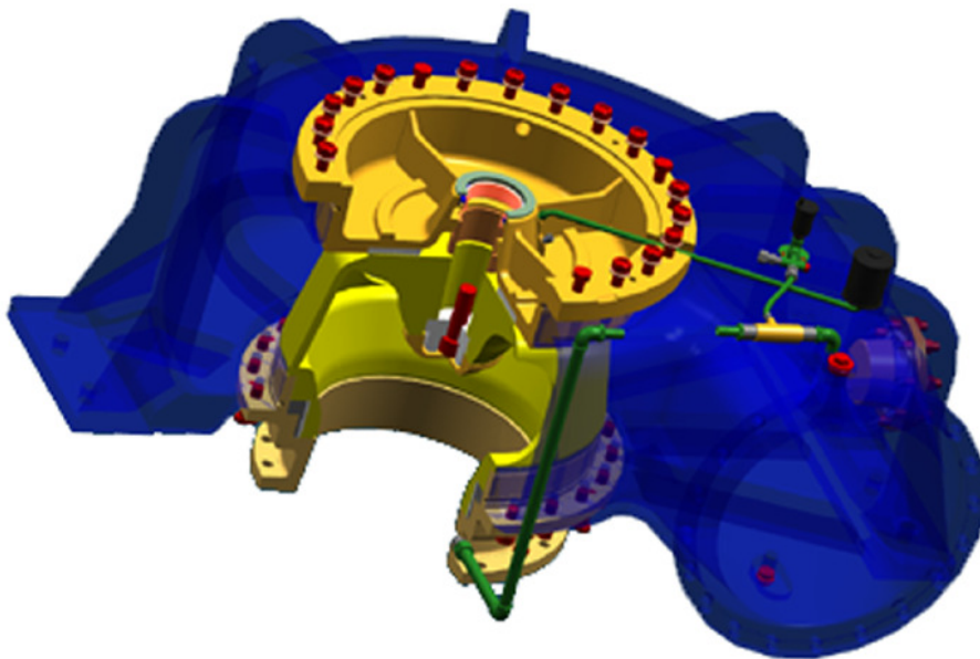
Das Bild zeigt: Spiralgehäuse mit Laufrad und Wellenabdichtung
