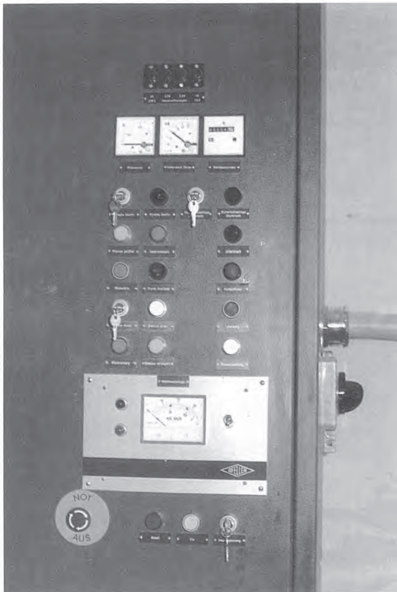
Bedienungspanel auf dem von uns gelieferten Schaltschrank. Unten Windmessanlage, oben Instrumente für Motorstrom, Überwachungsstrom und Betriebsstundenzähler.
