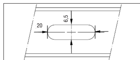
Langloch: an Plattentragprofil (Gleitpunkt)
