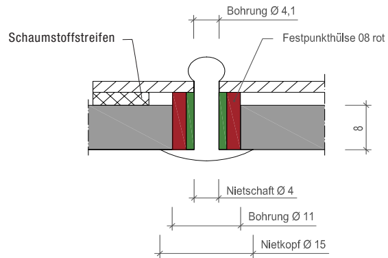
Festpunktausbildung
