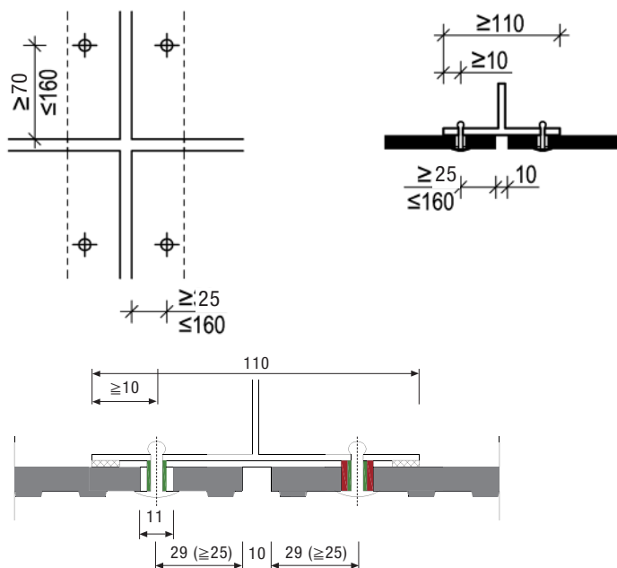
Plattenstoß bei vollem Plattenformat und Befestigung in der Achse des ersten Profilberges.
