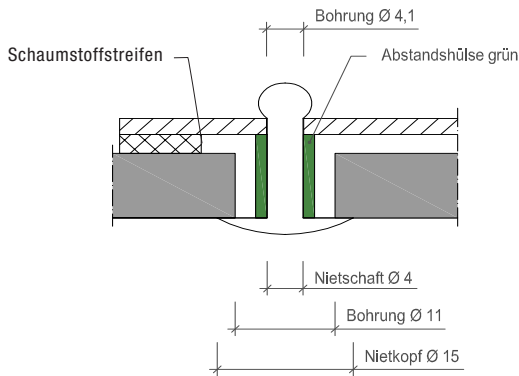
Gleitpunktausbildung
