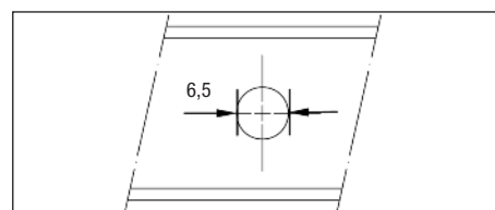
Rundloch: an Agraffe und Plattentragprofil (Festpunkt)
