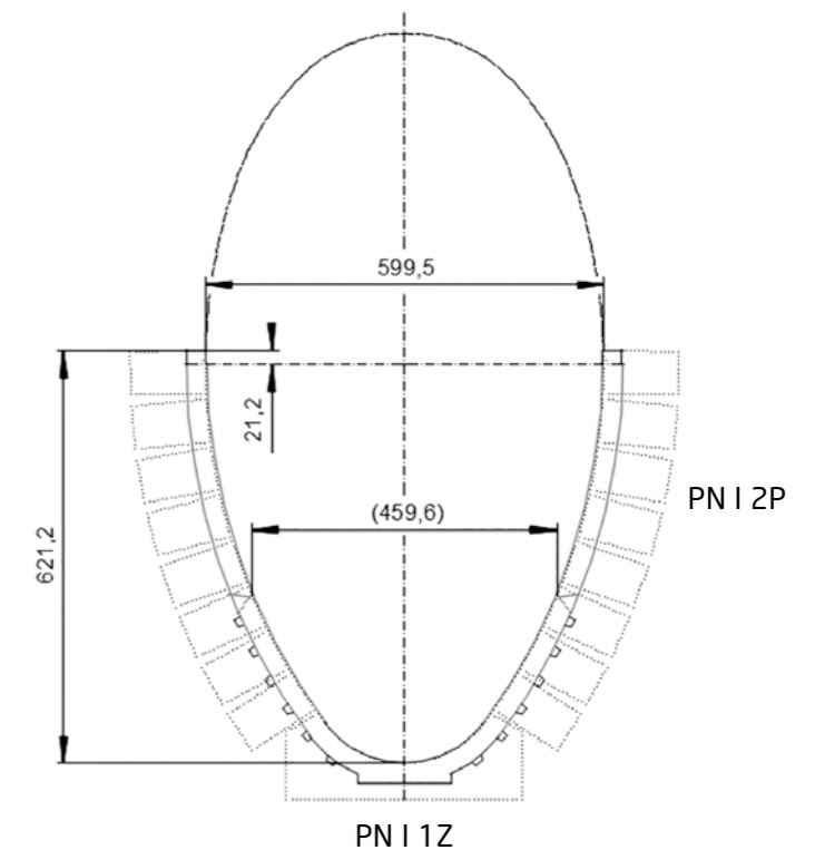
Beispiel: Kanalsole ausgekleidet mit einer Rinne und 2 Seitenteilen (jeweils mit einem Schloss)
