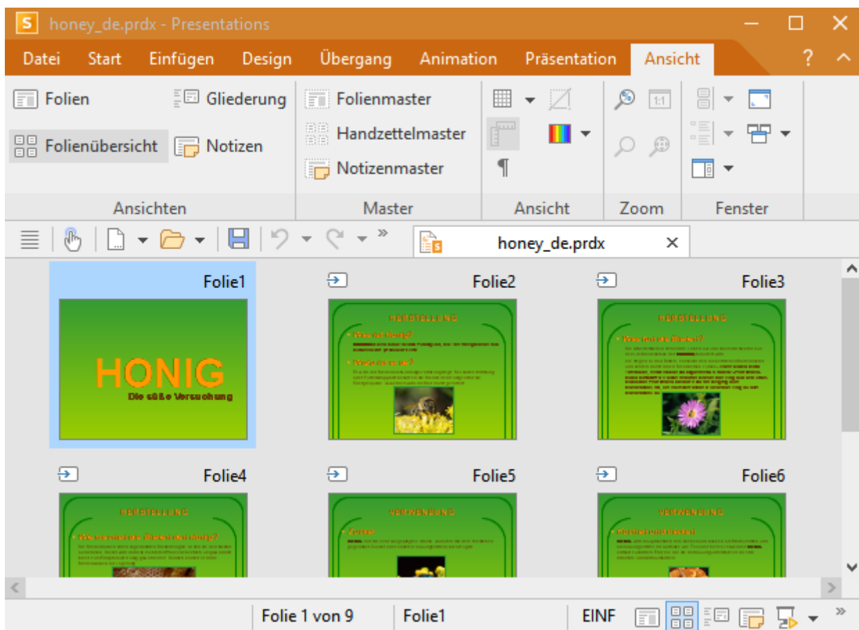
Die Folienübersicht
