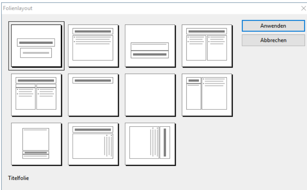
Der Folienlayout-Dialog
