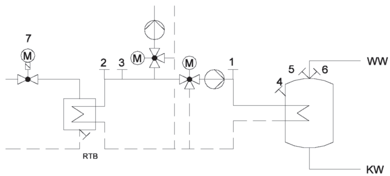
Bild 3: Anordnungsbeispiele
