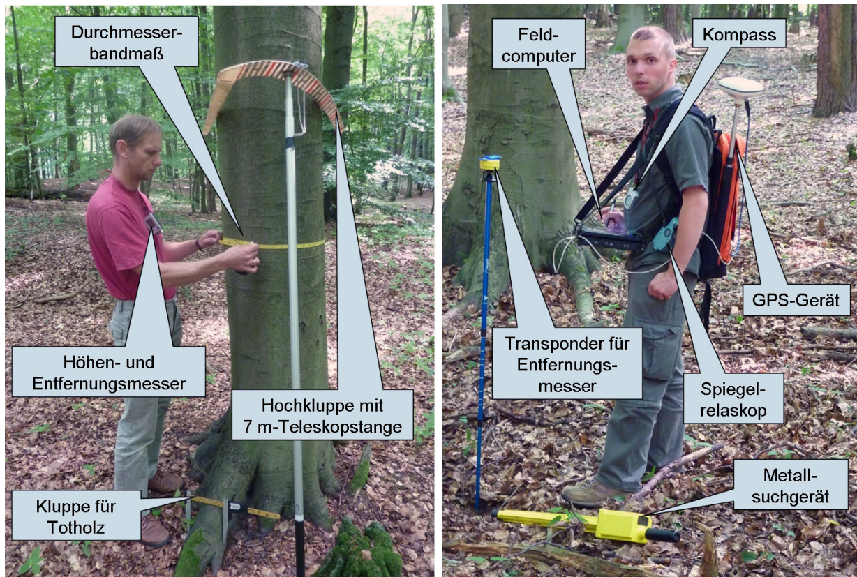
Abbildung 8: Arbeitsgeräte der Inventurtruppe
