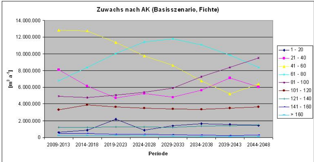
Abbildung C 7: Zuwachsentwicklung (Vfm) nach Altersklassen bei der Baumart Fichte
