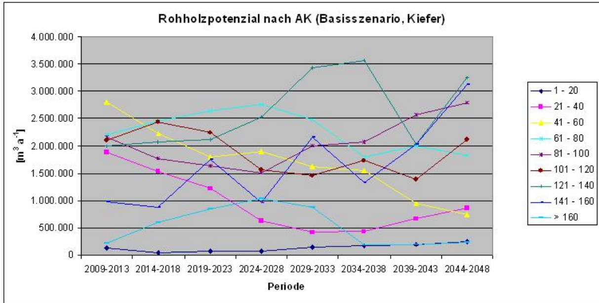
Abbildung C 12: Entwicklung des Rohholzpotenzials (Efm) nach Altersklassen bei der Baumart Kiefer
