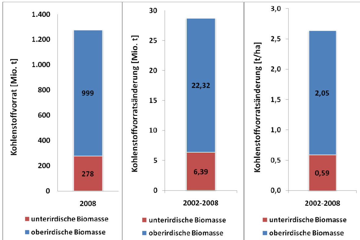
Abbildung 29: Kohlenstoffvorrat in der ober- und unterirdischen Biomasse für 2008 (links), Kohlenstoffvorratsänderung gesamt (Mitte) und pro Hektar (rechts) für den Zeitraum 2002 bis 2008
