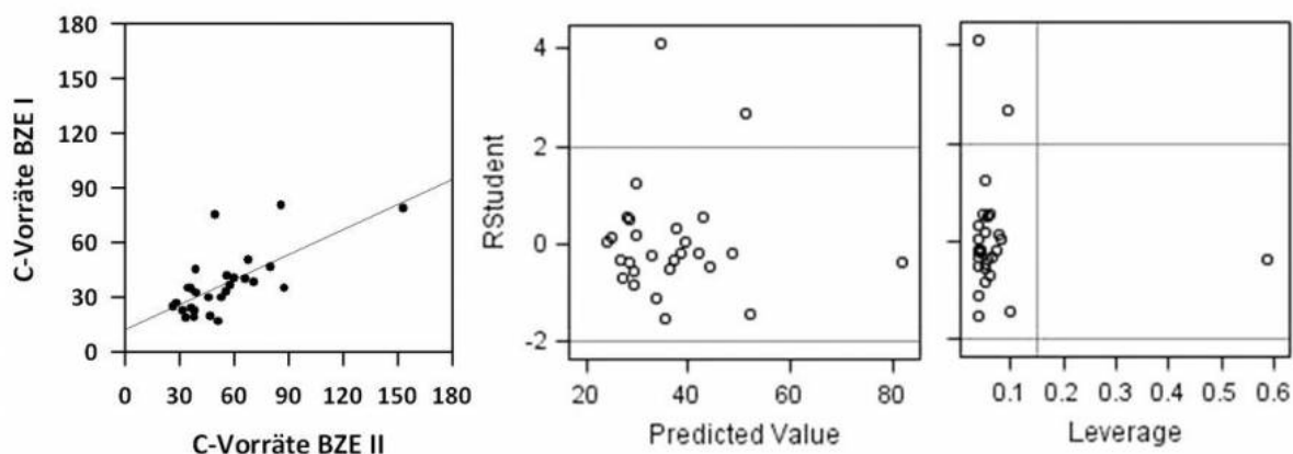
Abbildung 23: Regression zwischen C-Vorräten (0 - 30 cm) der BZE II/BioSoil- und BZE I- Daten (links) sowie die identifizierten Ausreißer anhand der Residuen-Analyse durch Student-Residuen (Mitte) und den "high leverage"-Punkten (rechts) am Beispiel der neu gebildeten Leitbodeneinheit Podsol-Parabraunerde / Podsol-Fahlerde / Fahlerde / Braunerde aus sandigen Deckschichten über Geschiebelehm
