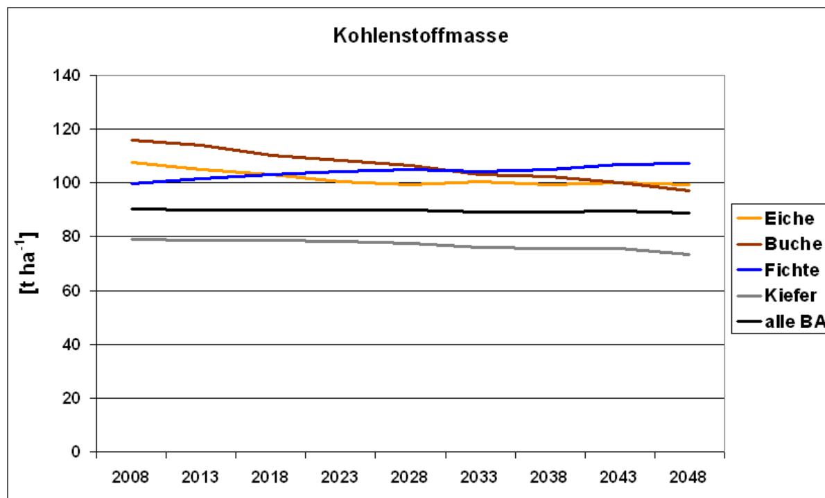
Abbildung 43: Durchschnittliche oberirdische Kohlenstoffspeicherung pro Hektar (tC)
