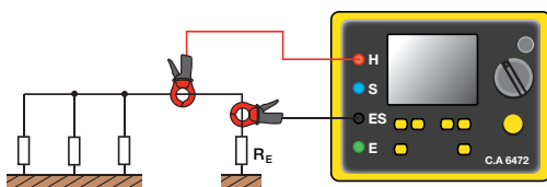
Prinzipdiagramm eines ausgedehnten Erdungsnetzes. In der Praxis besteht eine Erdung meist aus mehreren Basis-Schleifen, die ein ausgedehntes Erdungsnetz bilden.
