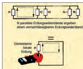
Prinzipdiagramm eines ausgedehnten Erdungsnetzes. In der Praxis besteht eine Erdung meist aus mehreren Basis-Schleifen, die ein ausgedehntes Erdungsnetz bilden.
