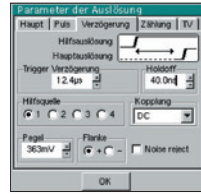
Die Effektivtriggerung für den Kanal erfolgt in diesem Beispiel mit einer Verzögerung von 12,4 µs gegenüber der Hilfsstromquelle.
