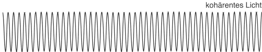
Bild 4.33: Modell für Licht aus klassischen Lichtquellen (oben und mitte) und stabilen Lasern (unten). Der obere Fall soll das Licht einer spektral breiten, der mittlere einer monochromatischen klassischen Lichtquelle demonstrieren.
