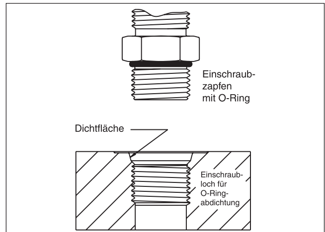
Abb. 5 – UNF-Einschraubgewinde
