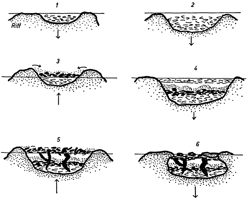
Abb. 1: Sedimentationsablauf der bunten Rhät-Lumachelle im Adnetter Kirchenbruch
