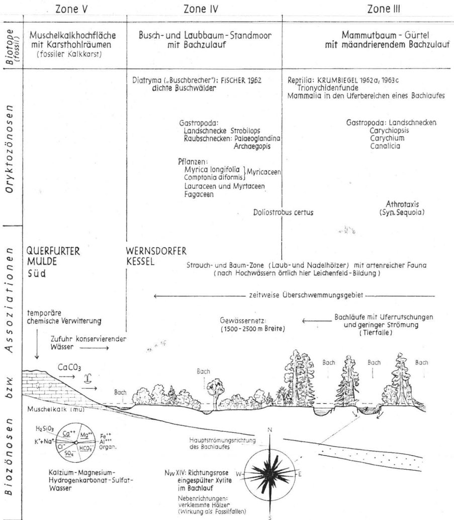
Abb. 5. Rekonstruktion der fossilen Pflanzen- und Tiergesellschaften (fossile Biozönosen) in ihrer seitlichen Aufeinanderfolge in den Lebensbereichen der Trichtertümpel Neumark-Süd N S XXII und N S XX (Fundstellentyp: Einsturztrichter-Einbruchstyp, Setzungstyp/Bach-
