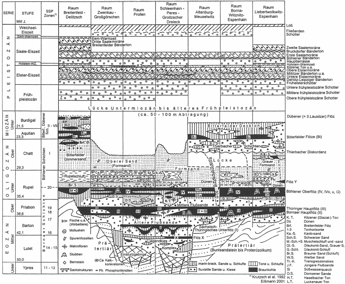
Abb. 1. Quartär (stark vereinfacht) und Tertiär wichtiger durch Braunkohlentagebau erschlossener Sektionen der mittleren und südlichen („Weißelsterbecken“) Leipziger Tieflandsbucht.
