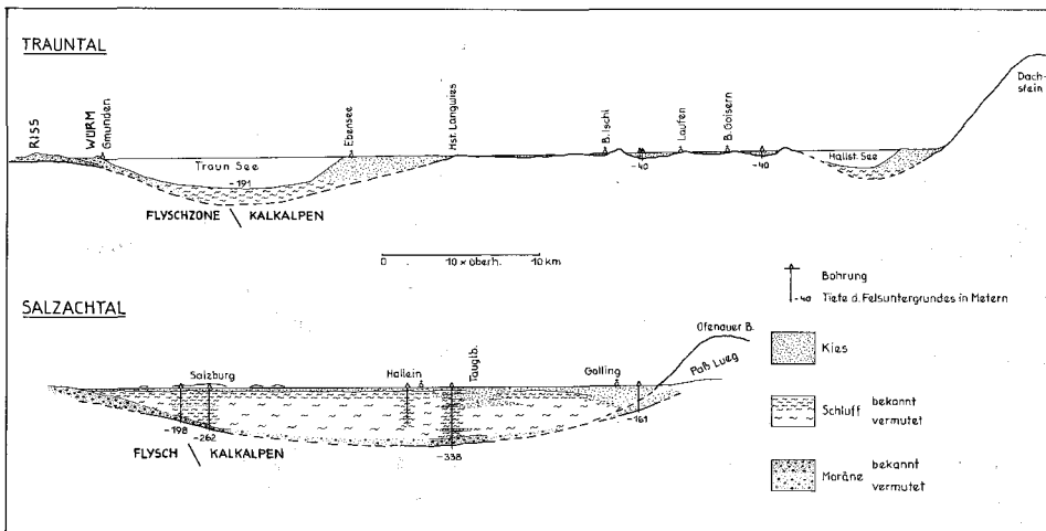
Abb. 1: Übertiefte Becken
