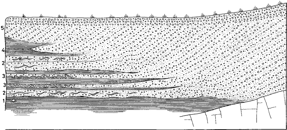
Abb. 5: Schematische Darstellung der Sedimente und Strukturen in einem Eisrandtausee mit hoher Sedimentationsrate.
