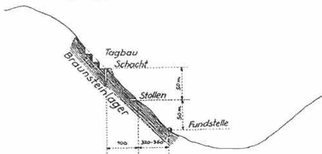
Fig. II Ideelles Längsprofil nach G - B
