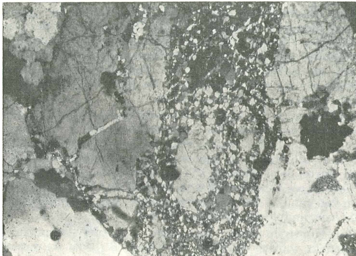
Abb. 5. Granittypus A/a (Nicols \perp ). Mörtelquarze als Kluffüllung in Kalifeldspathoporphroblasten.
