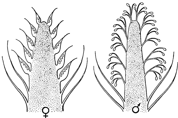
Abb. 3 .Urangeospermen-Blüten, wie sie etwa im frühen Mesozoikum existiert haben. Sie waren eingeschlechtig, windblütig und hatten zahlreiche Blütenorgane.
