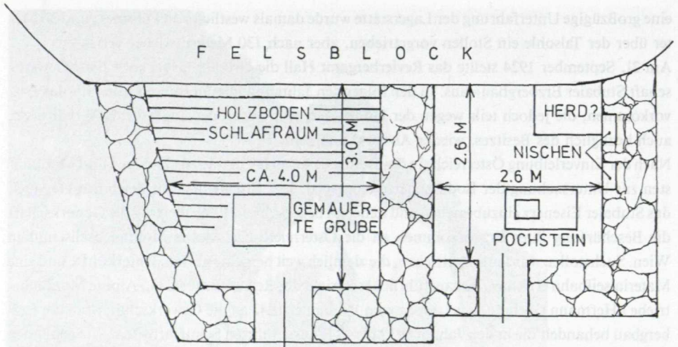
Die Knappenhütte am Glücksgrat. Zustand der Ruine im Jahre 1982. Zeichnung von Helmut Leutelt.
