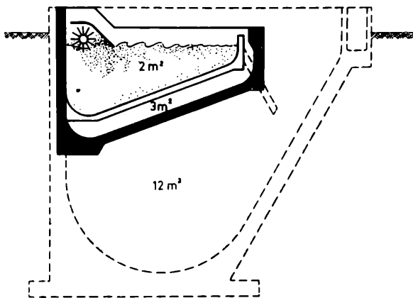
Abb. 18. Belebtschlammbecken nach TNO — Dr. Pasveer und frühere Form
