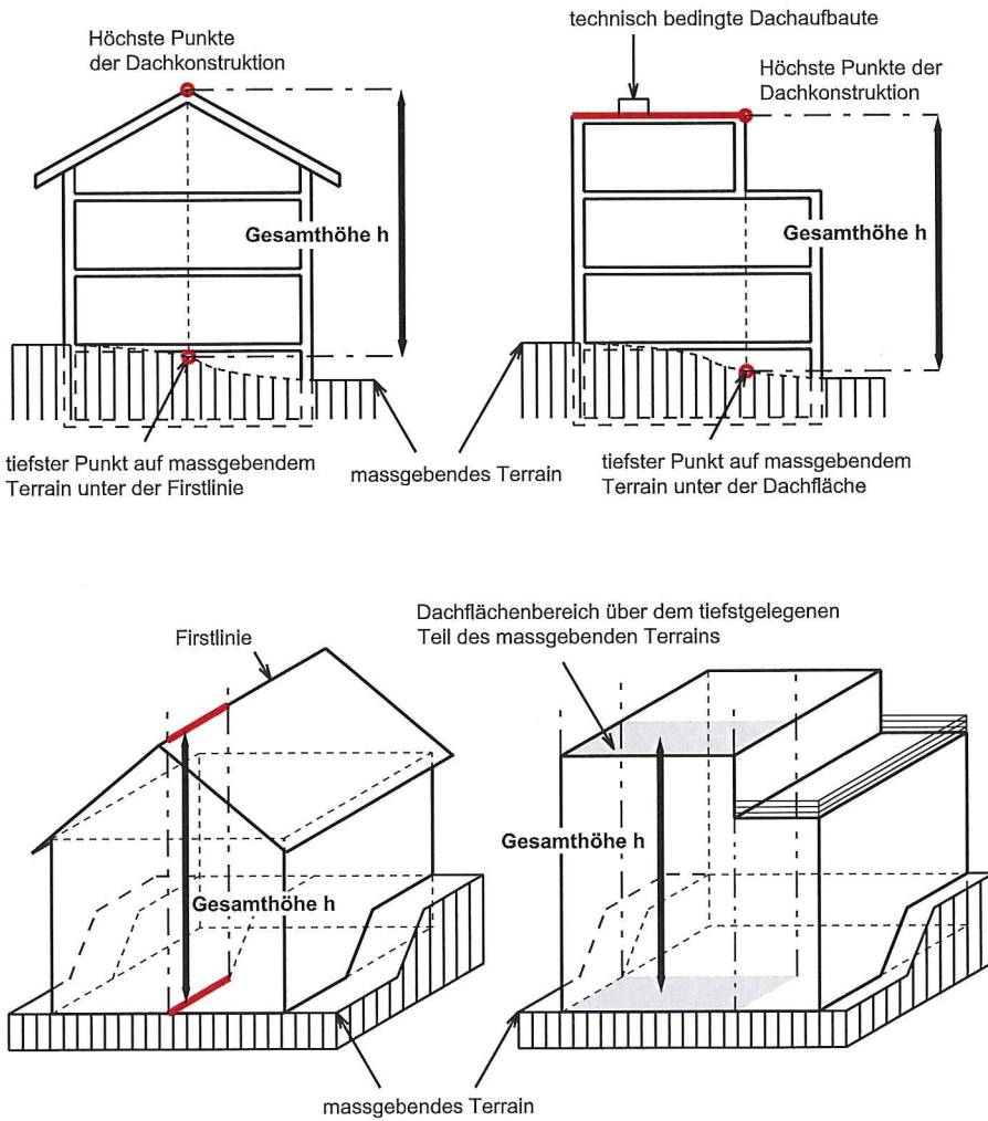
Figur 5.1 Gesamthöhe
