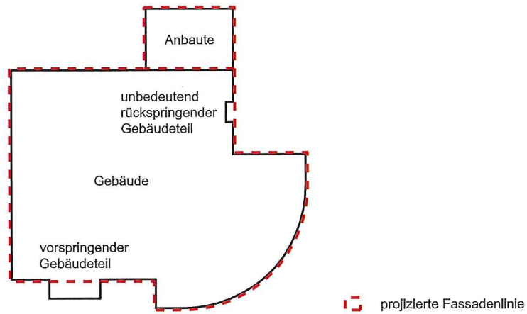
Figur 3.3 Projizierte Fassadenlinie
