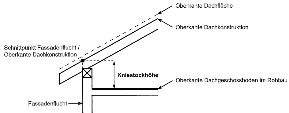
Figur 5.3 Kniestockhöhe
