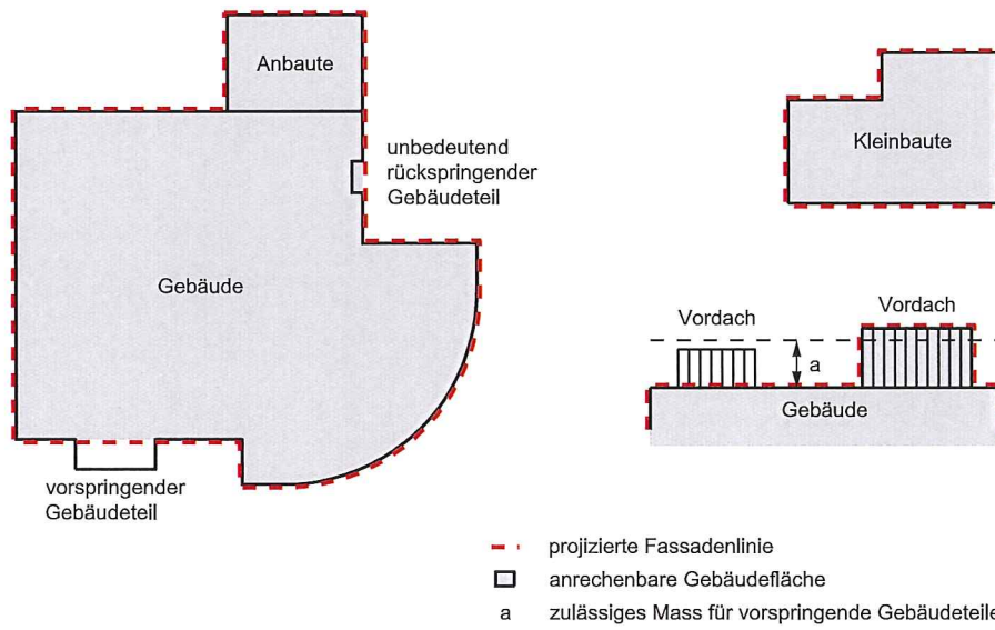
Figur 8.4 Anrechenbare Gebäudefläche
