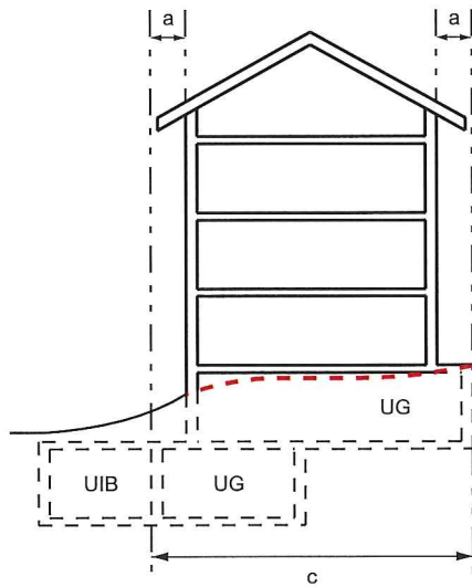
Figur 6.2 Untergeschosse
