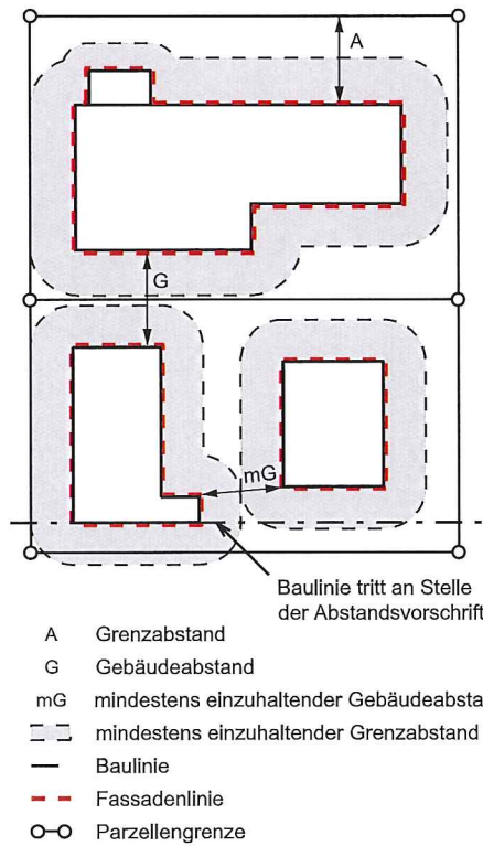
Figur 7.1 - 7.3 Abstände und Abstandsbereiche
