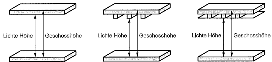
Figur 5.4 Lichte Höhe
