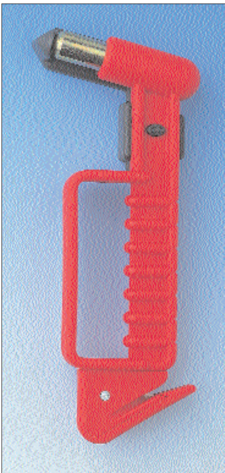
274 0043 Nothammer mit Gurtschneider inkl. Halterung PP, rot / POM, grau Stahleinlage: verz., gelb passiviert Spitze: Hartmetall 260 g/St. VE 1 St.
