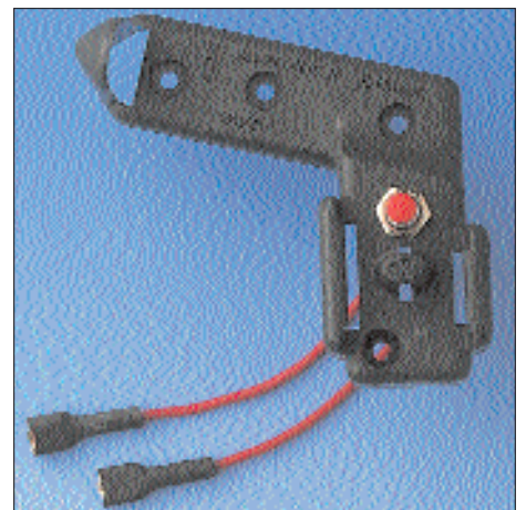
274 0039 Nothammerhalterung zu 274 0037 / 0045 mit Drucktaster und Kabel zur Signalauslösung POM, grau 40 g/St. VE 10 St.
