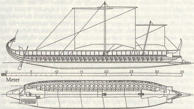
Zeichnung einer attischen Triere
