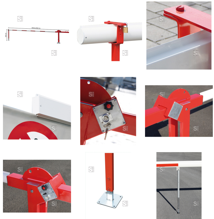
Anwendungsbeispiel: Wegesperre mit Gegengewicht -Alpha 150- in rot-weiß/reflex (Art. 13698-030301)
