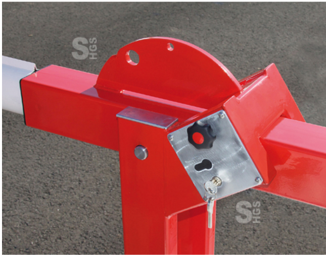
Detailansicht: ... zum Umbau der Schlösser von links nach rechts
