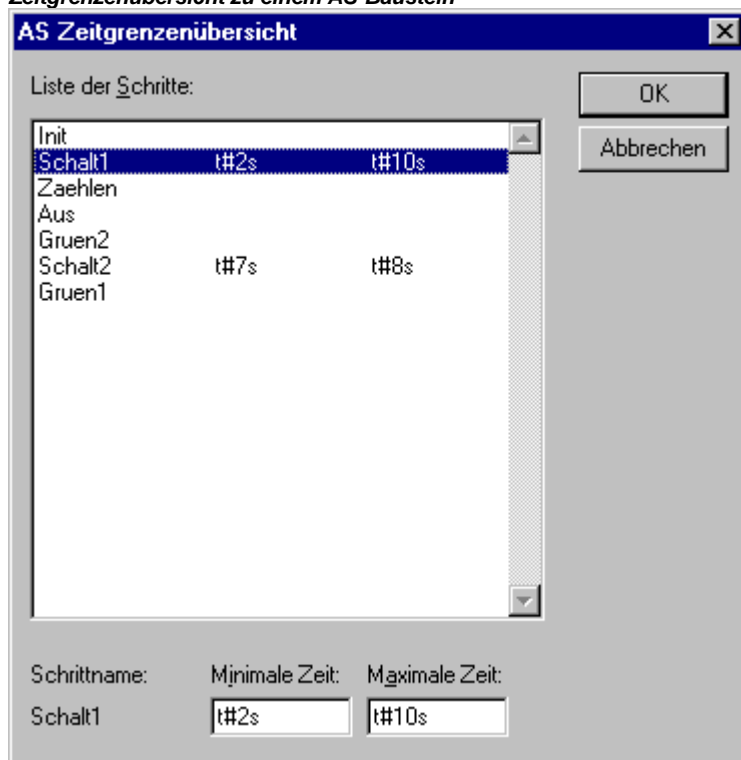
Zeitgrenzenübersicht zu einem AS-Baustein
