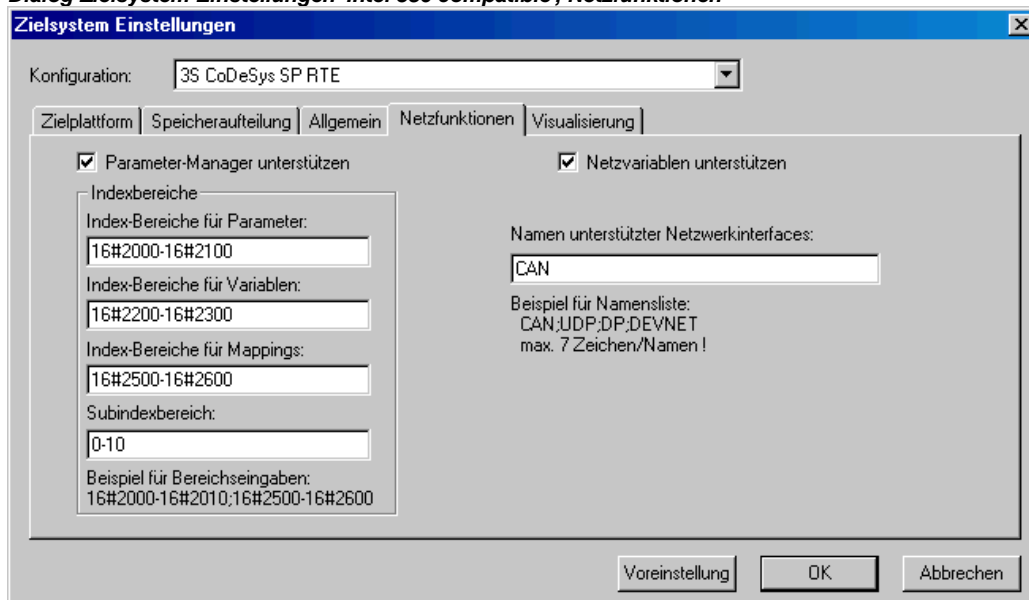
Dialog Zielsystem Einstellungen 'Intel 386 compatible', Netzfunktionen
