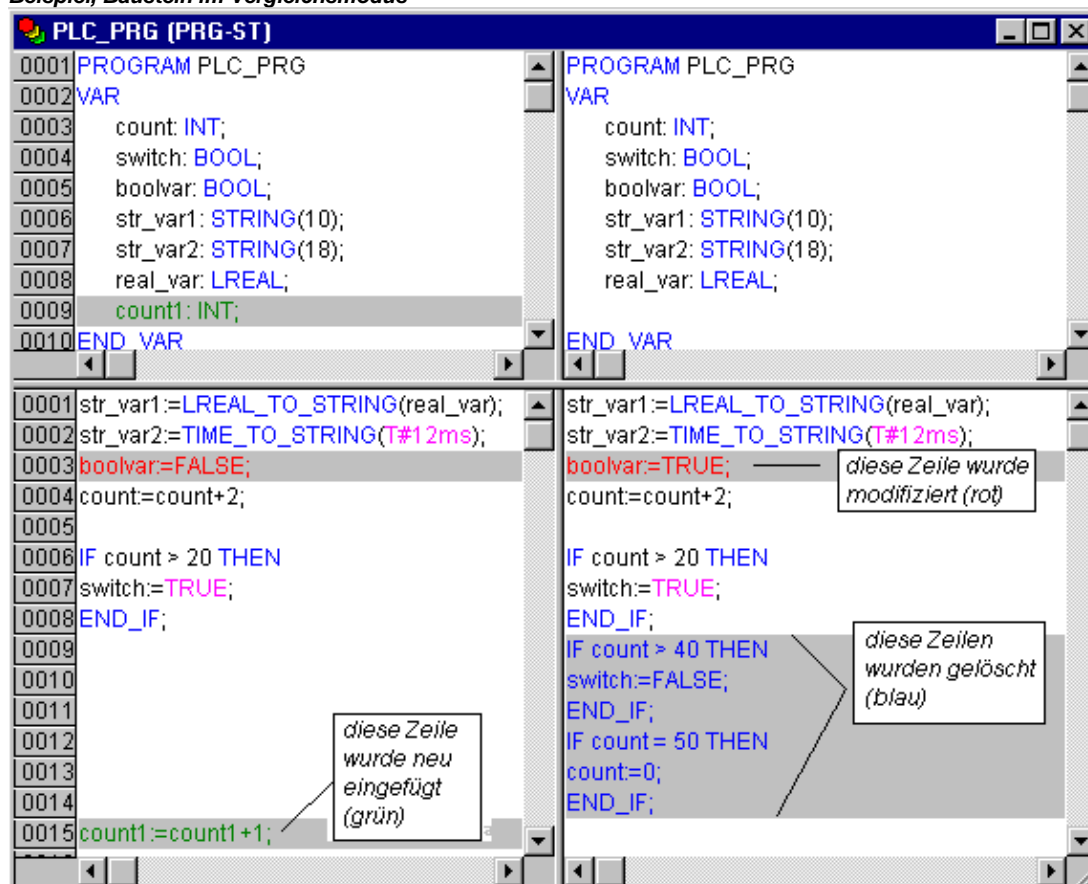
Beispiel, Baustein im Vergleichsmodus
