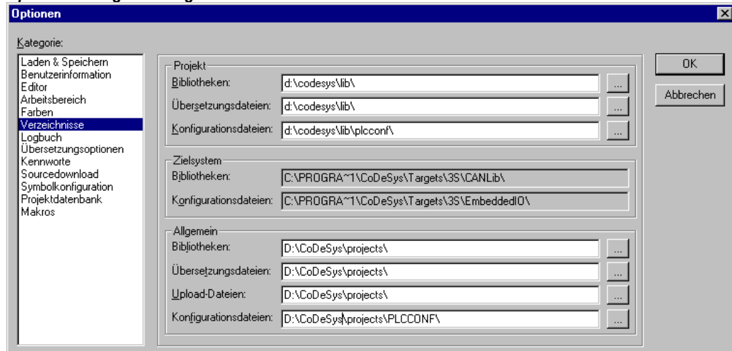
Optionen-Dialog der Kategorie Verzeichnisse
