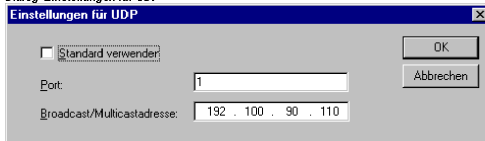
Dialog 'Einstellungen für UDP'
