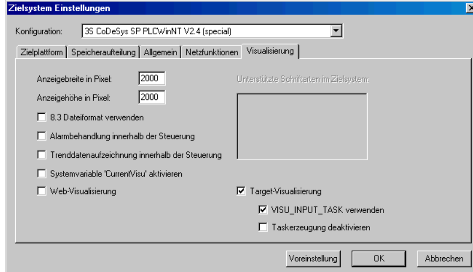
Dialog Zielsystem Einstellungen 'Intel 386 compatible', Visualisierung
