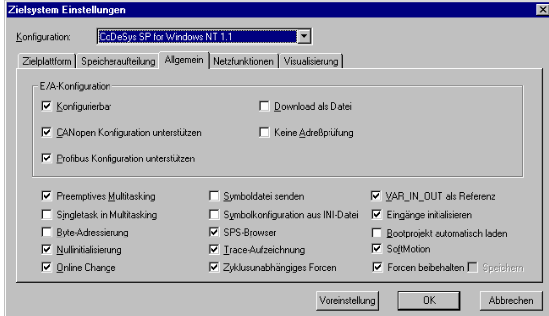
Dialog Zielsystem Einstellungen, Allgemein
