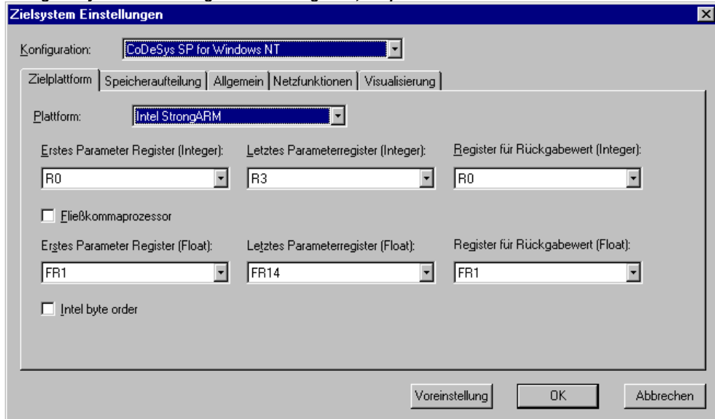
Dialog Zielsystem Einstellungen 'Intel StrongARM', Zielplattform
