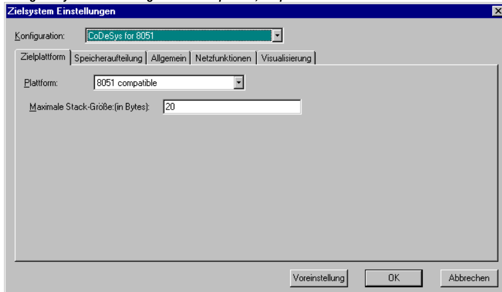
Dialog Zielsystem Einstellungen '8051 compatible', Zielplattform
