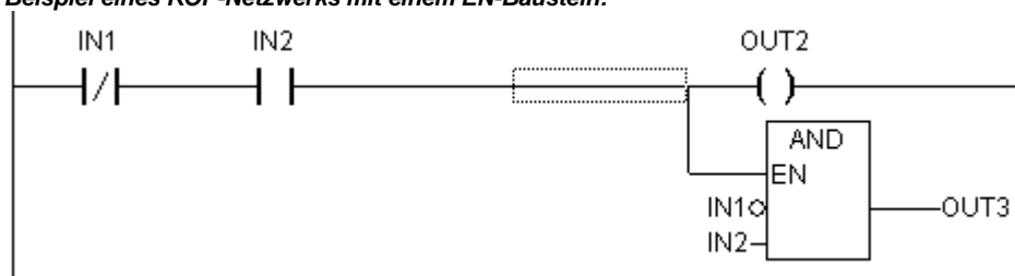
Beispiel eines KOP-Netzwerks mit einem EN-Baustein:
