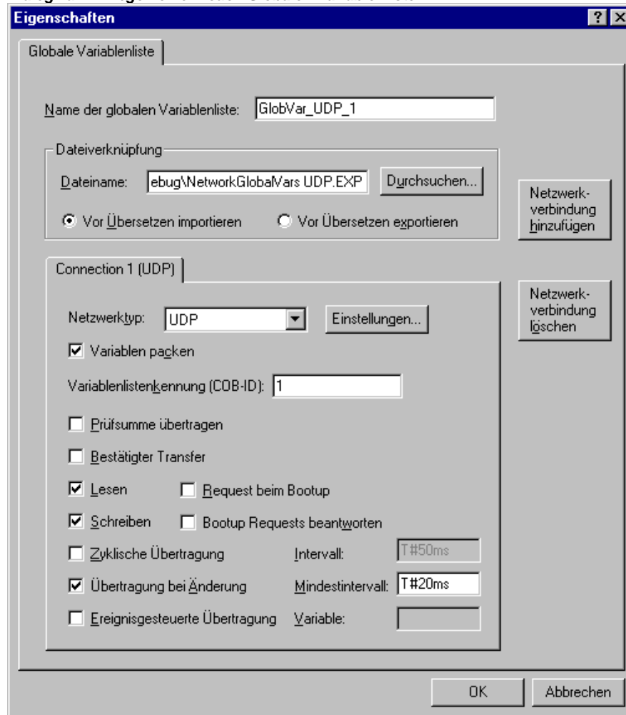
Dialog zum Anlegen einer neuen Globalen Variablenliste
