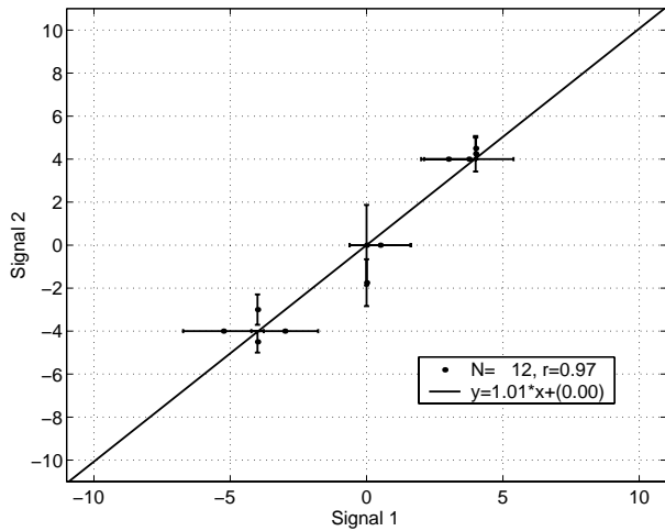
Abbildung 1: Verstärkung der 1. Blockharmonischen zweier Originalsignale, so dass beide Geräusche gleich starkes Profilgeräusch enthalten.
