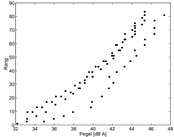
Abbildung 2: Rang entsprechend der Stärke des Profilgeräuschs (höherer Rang entspricht mehr Profilgeräusch) in Abhängigkeit vom Pegel (Wurzel des zweiten Moments) der 1. Blockharmonischen.
