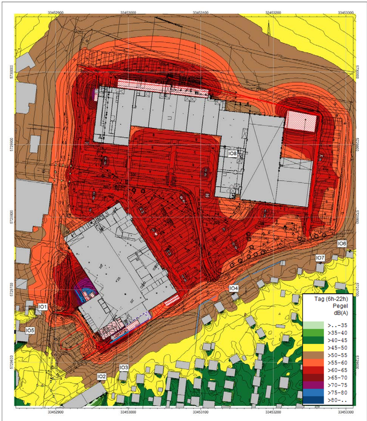
Bild 1 Schallimmissionsraster Beurteilungspegel, Gewerbelärm Tag, Nachweisebene 6 m
