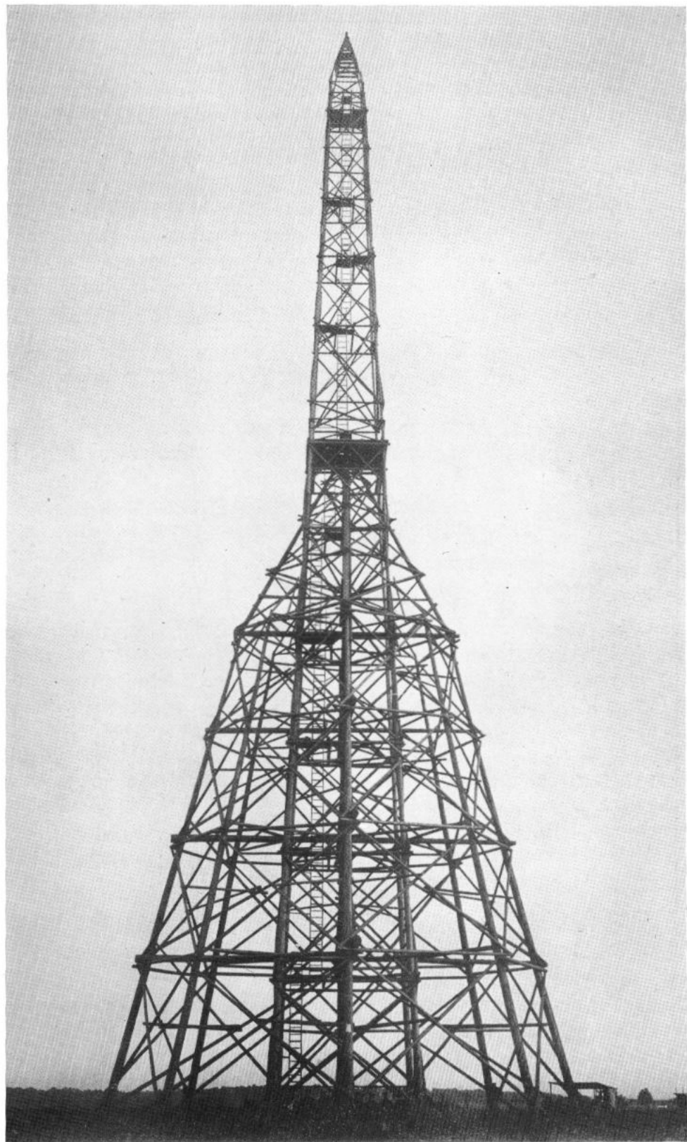
Abb. 2: Hölzerner Signal- und Beobachtungsturm für die Triangulation I. Ordnung (Gesamthöhe 60 m)
