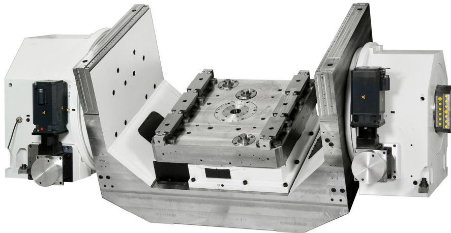
2 Achs - NC Rundtisch Kombination FIBROPLAN mit Paletten – Spann – System
