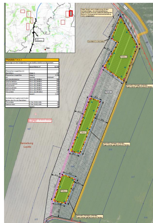
Ausschnitt Ausführungsplan für die Maßnahmen T-A 4.1 und T-A 6.1 im Bereich Mauschwitz
