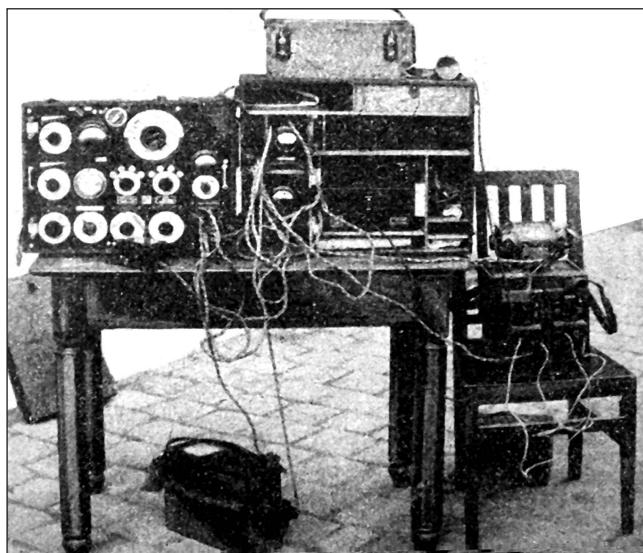
9. ábra. A kép aláírása: 10 W kisorádió-állomás (Magyar Katonai Zsebkönyv 1928)
