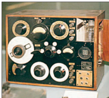
6. ábra. Az ARS 69 (Milánó, Technikai Múzeum, a szerző felvétele)
