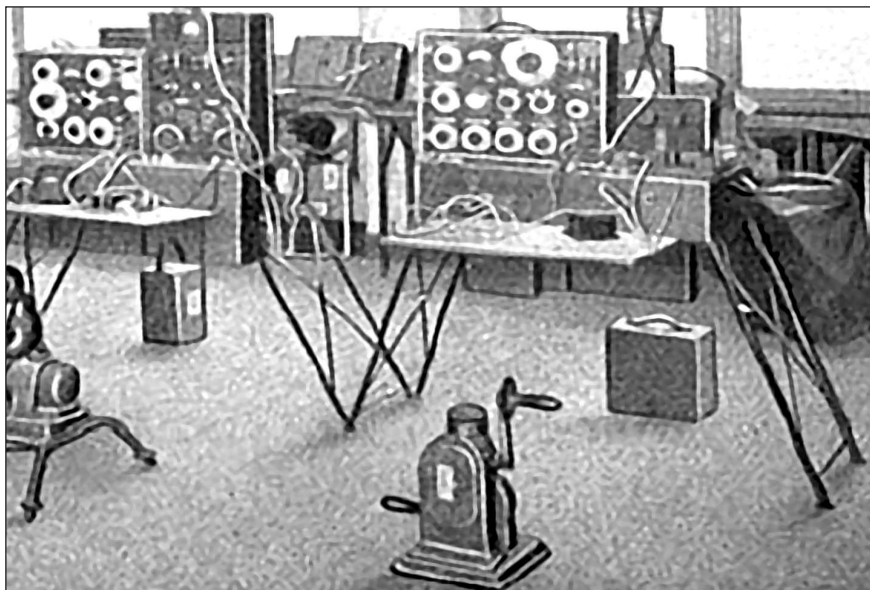
5. ábra. Részlet a Telefunken mintateremből, jobbra az ARS 68 (Telefunken Zeitung)
