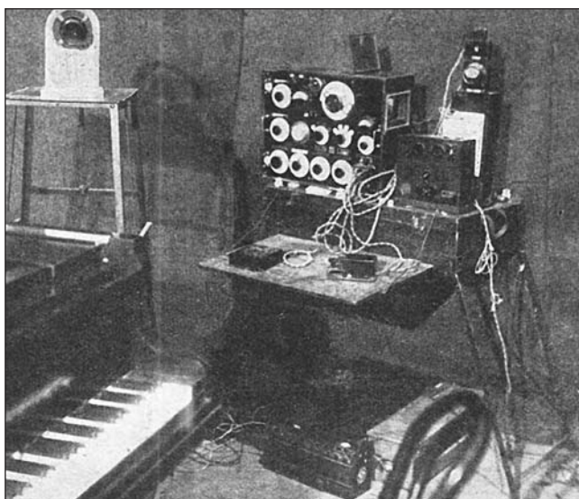
8. ábra. A miskolci Vegyesdandár egyik készüléke a miskolci Rádiókiállításon 1927-ben
