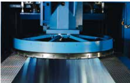
Fräsen mit 3'100mm-Messerkopf
