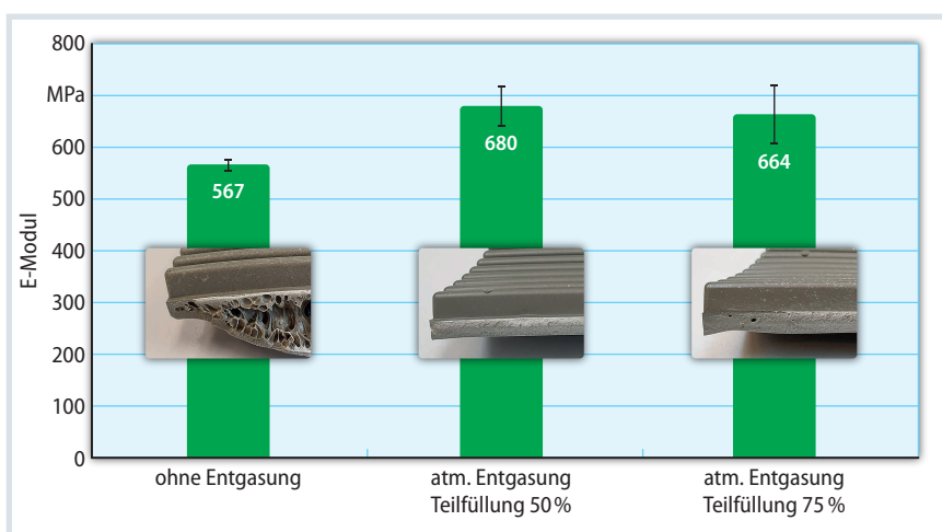
Bild 3. Die Bauteilqualität ist abhängig von der Entgasung und dem Füllgrad der Einspritzschnecke. Ohne Entgasung weist das Musterteil sehr große Poren auf. Das Bild zeigt die E-Modul aus der Versuchsreihe mit PP-Folienagglomerat. Quelle: Engel; Grafik: © Hanser
